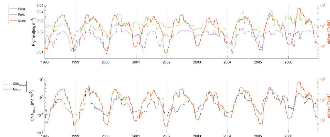
Figure IV.5: Série temporelle de comptage in-situ de Micro, vis-à-vis des différents pigments secondaires (a) et de la Chla Micro (b) au niveau de la station du Golfe de Naples.
