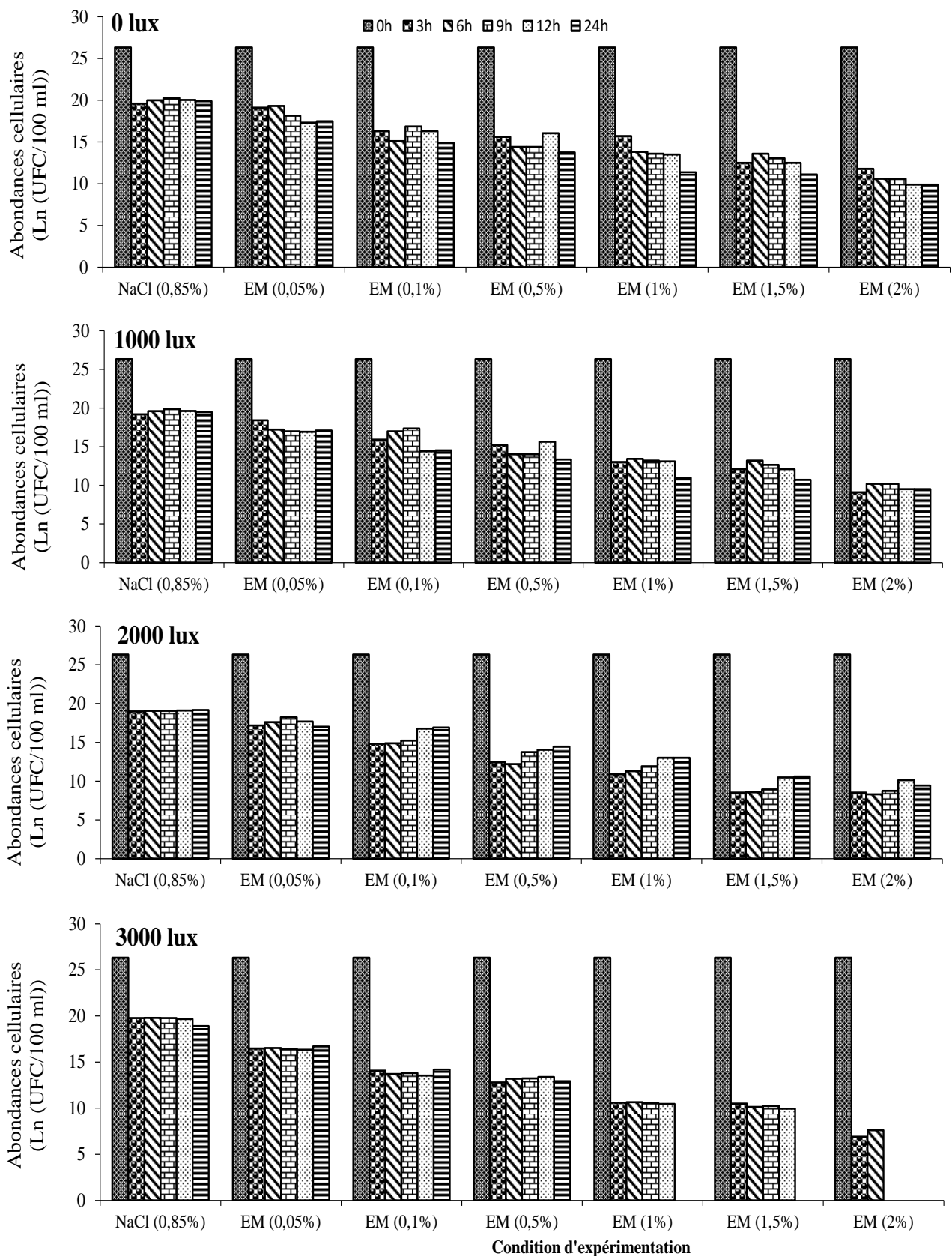
Figure 31: Variation temporelle des abondances cellulaires d' Enterococcus faecalis en présence de différentes concentrations d'extrait d' Eucalyptus microcorys (EM) sous différentes intensités lumineuses.
