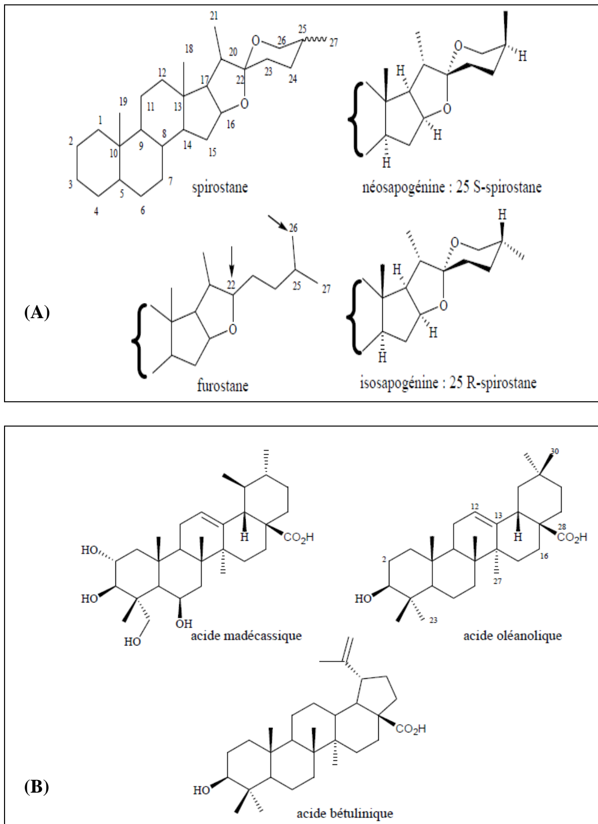
Figure 6: Squelettes et configurations des génines stéroïdiques des saponosides (A) et exemples de génines triterpéniques (B) (Bruneton, 2009)
