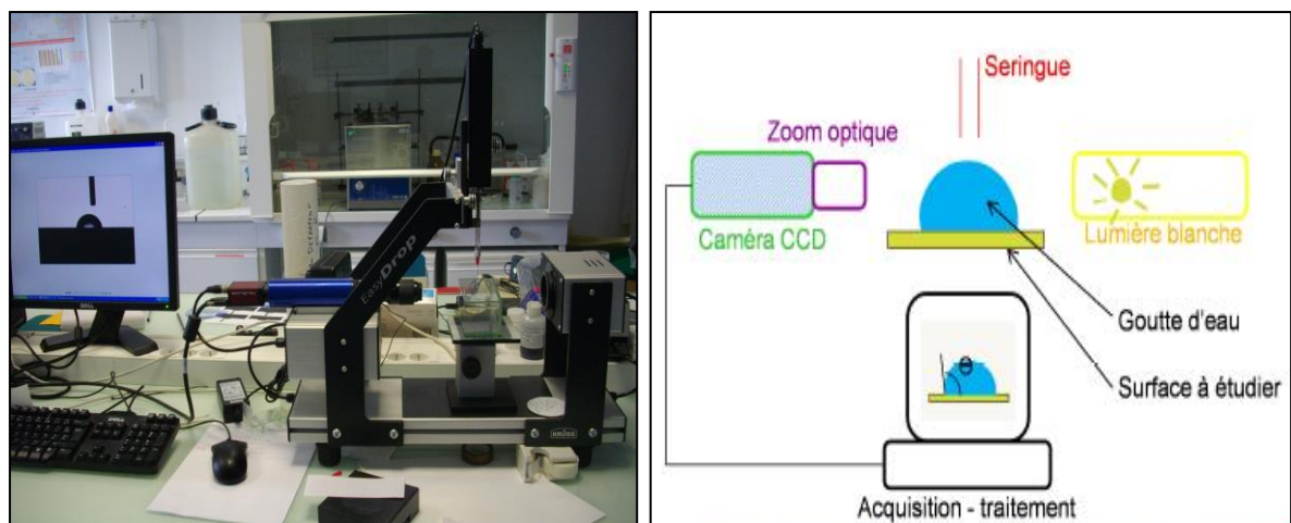
Figure 19 : Appareil de mesure des angles de contact : Goniomètre de marque « Krüss », modèle « Easy Drop ».
