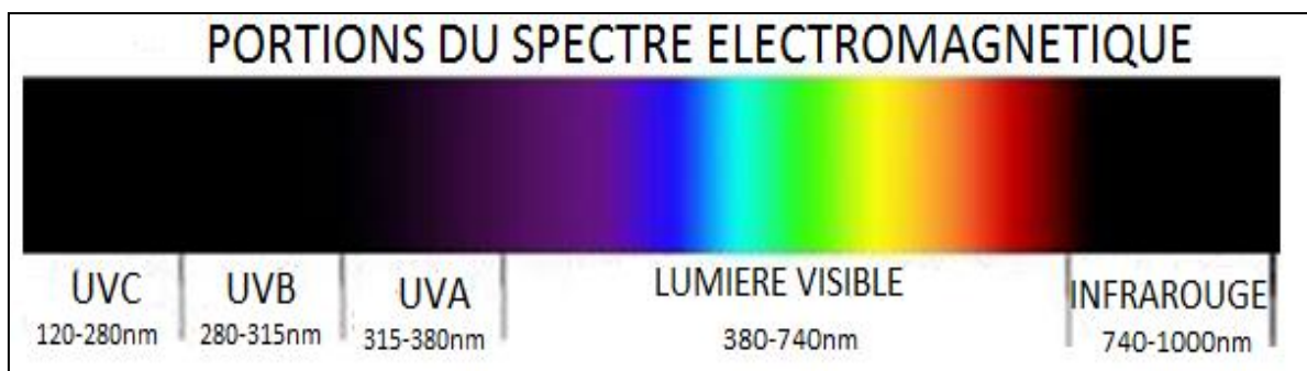
Figure 10 : Différentes portions du spectre électromagnétique (Downes et Blunt, 1877)
