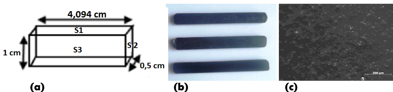
Figure 15 : Représentation graphique (a), photographie (b) et microscopie électronique à balayage (c) du polyéthylène.
