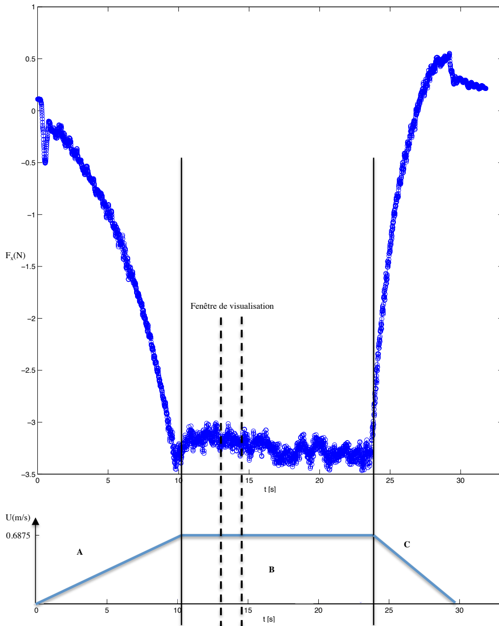
FIGURE 2.9 – Comparaison de l'évolution de l'effort de traînée avec la vitesse du chariot de traction en fonction du temps. Exemple du cylindre de diamètre D = 8 cm avec un Re = 55\,000 correspondant à un Fr \simeq 0.78 .
