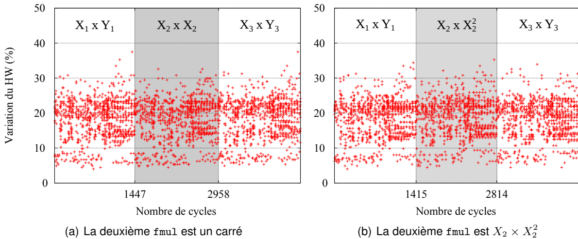
FIGURE 6.16 – Trois fmul avec différents types d'opérandes
