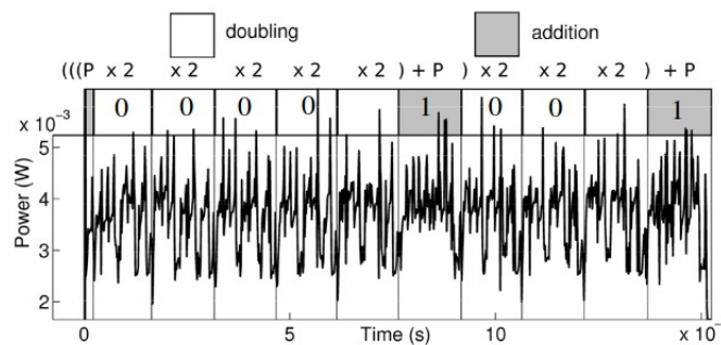
FIGURE 2.3 – Trace d'un doublement et addition [98]
