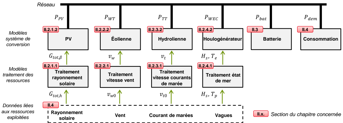
Figure II-1 : Vue globale du modèle du système multi-sources considéré et sections du chapitre concernées
