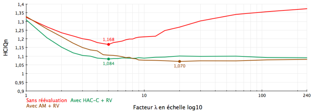
FIGURE 5.14 HClQ n de la méthode AM + RV et de la méthode HAC-C + RV en fonction de divers seuils λ du regroupement mono-gaussien/BIC pour les corpus ESTER 1, ESTER 2, ETAPE et REPERE 1 regroupés
