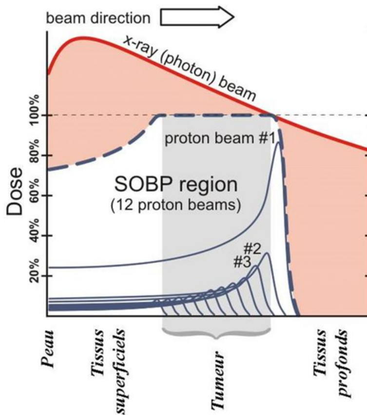
Figure 3 : Dans un plan de traitement typique pour l'hadronthérapie, le pic de Bragg étalé (SOBP : spread out Bragg peak), ligne pointillée bleue, est la distribution de rayonnement thérapeutique.
