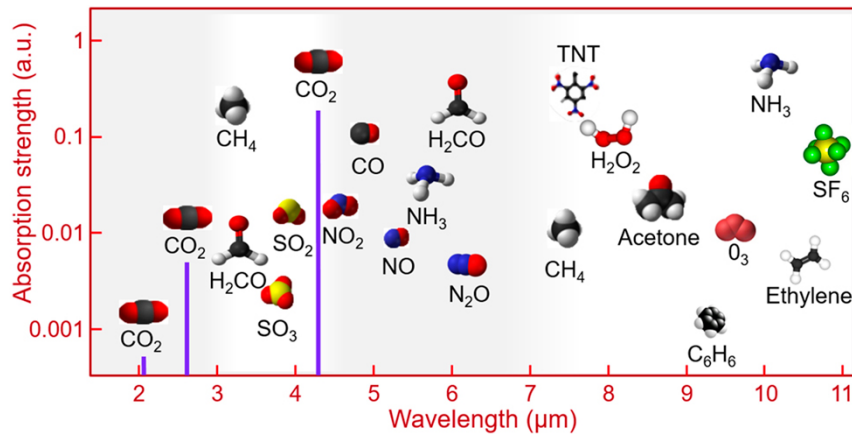
FIGURE I.9 – Représentation de la position spectrale des pics d'absorption dans l'infrarouge de différentes molécules (Mirphab).
