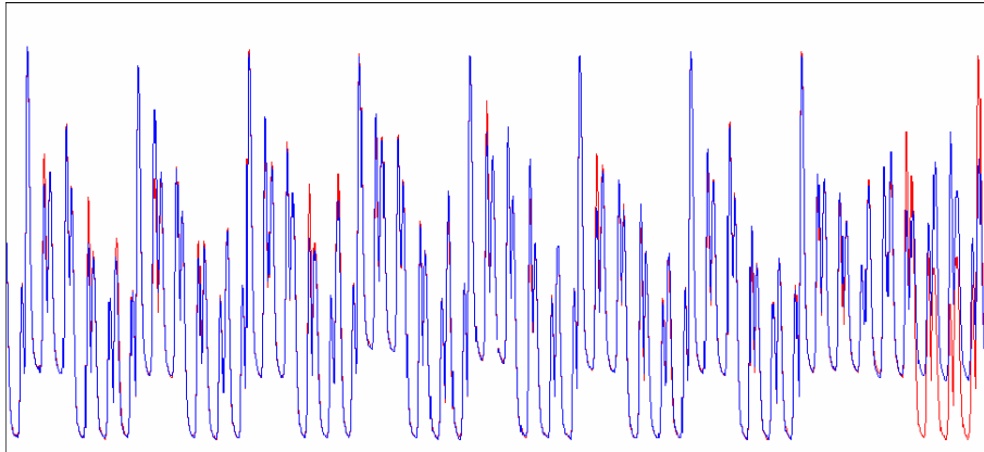
FIG. 1.11 – La consommation de courant dépend des instructions exécutées.
