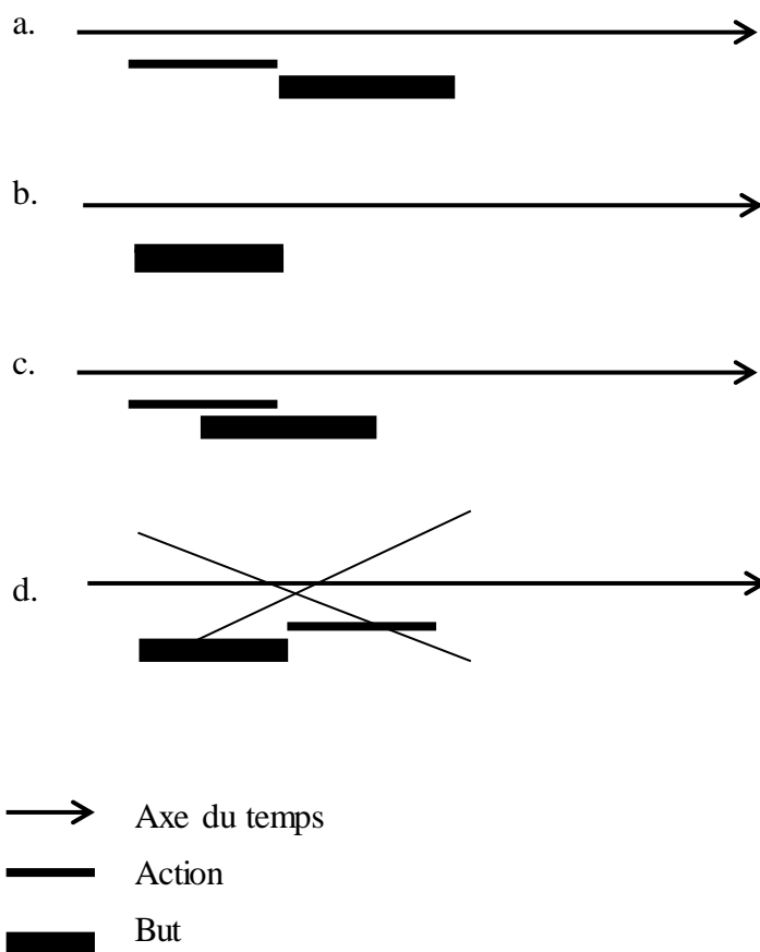
Figure I : relations temporelles dans la CVS à relation finale 63
