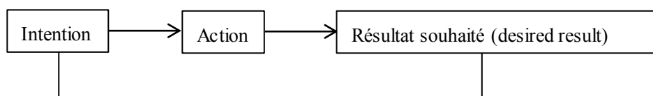
Figure III : la structure conceptuelle des buts (Schmidtke-Bode 2009 : 19)
