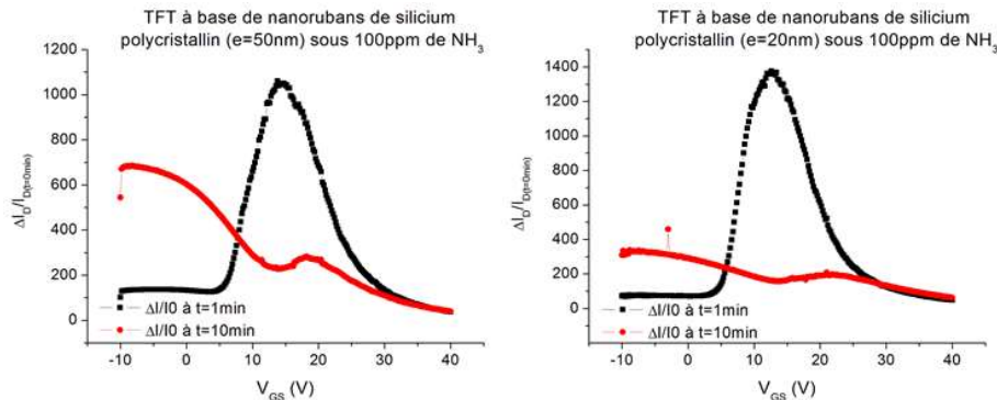
Figure 21: Variation relative du courant sous flux NH_3/N_2 en fonction de la polarisation de grille
