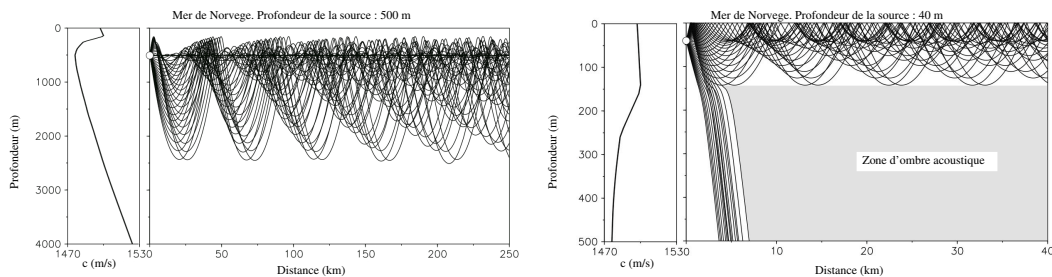
FIGURE 2.5 – Illustrations tirées de Computational Ocean Acoustics (Jensen et al. 2011 [59]). A gauche, un effet de canal à grande profondeur de type SOFAR. A droite, un profil particulier dû aux eaux froides et douces de surface créant un canal peu profond, ainsi que des zones d’ombre acoustique où la propagation est pratiquement nulle. Simulation pour une source émettant à des fréquences de l’ordre du kilohertz.
