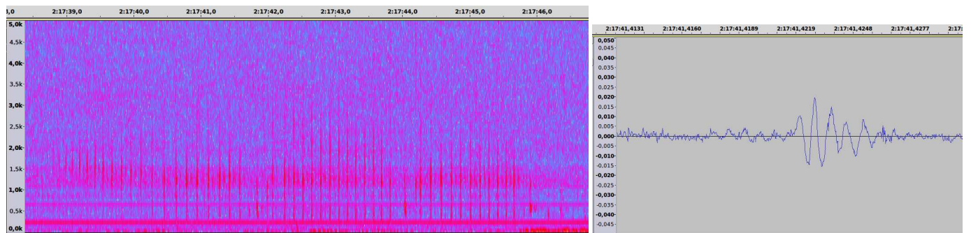
Figure 1: Sons brefs basse fréquence, fichier 170206_03 de 2h17min38 à 2h17min48, audacity, FFT de 1024 points, fenêtre Blackman (à gauche) Zoom, en forme d'onde, sur un son bref basse fréquence, fichier 170206_03 autour de 2h17min41.42s (à droite)
