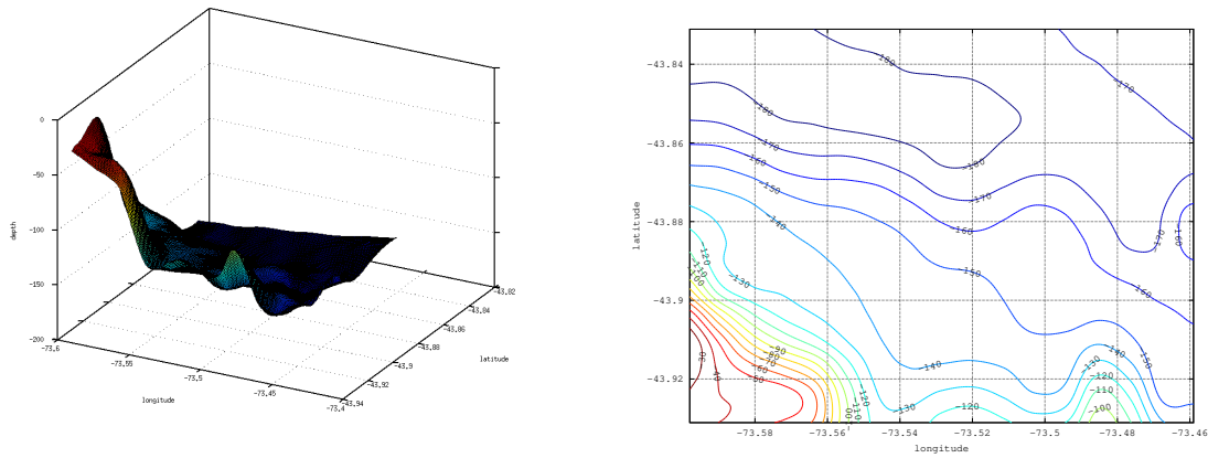
FIGURE 6.3 – Bathymétrie de la zone de Corcovado où est construit le premier modèle, tirée du site de données publiques GMRT [52]. A gauche, une vue en trois dimension et à droite, les lignes isobathes. L’hydrophone est placé au centre de la boîte, à 10 mètres du fond.
