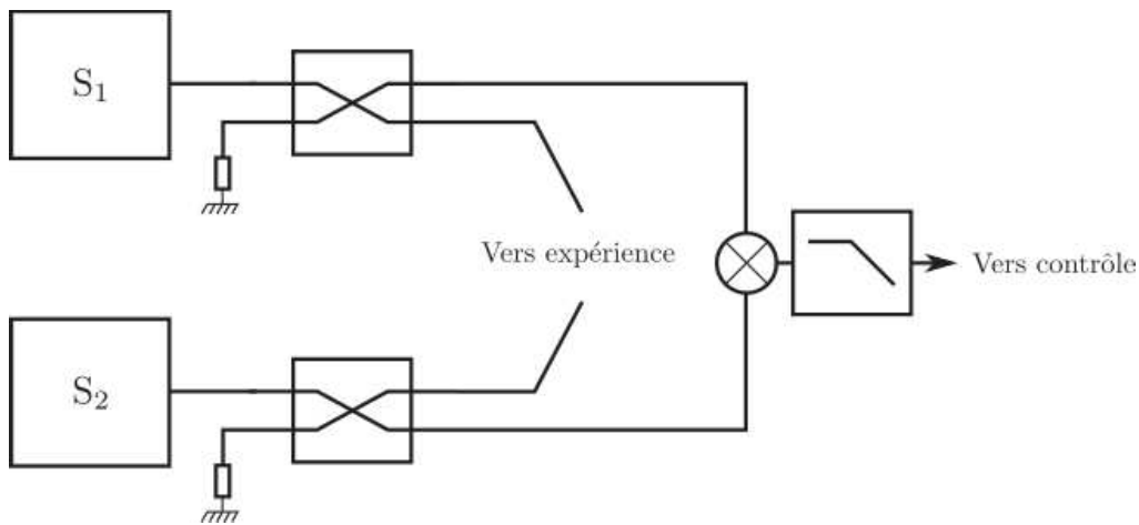
Fig. I.32 Schéma de principe du circuit utilisé pour les injections micro-onde. Les champs produits par les sources S_1 et S_2 sont divisés en deux. Une partie va vers l'expérience, tandis que l'autre va vers un multiplicateur où les deux signaux sont mélangés. Le battement obtenu est filtré pour garder la composante basse fréquence qu'on envoie vers l'ordinateur de contrôle de l'expérience afin de déclencher la séquence expérimentale pour une phase relative donnée des deux injections.
