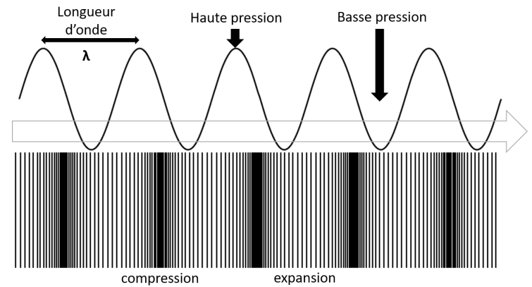
FIGURE 1.21 – Illustration d'une onde sonore se propageant. La pression varie cycliquement comme une onde sinusoïdale (haut); déplacement des particules en déphasage par rapport à la pression (bas). Figure inspirée de Simmonds & MacLennan [2005].
