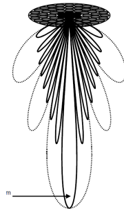
FIGURE 1.22 – Exemple de représentation tridimensionnel d'un faisceau : le lobe principal du centre (indiqué par une flèche) a la plus grande énergie acoustique et cette énergie décroît au fur et à mesure que l'on s'éloigne du lobe principal. Plus la surface d'émission est grande, plus le faisceau est étroit. Figure extraite de Simmonds & MacLennan [2005] .
