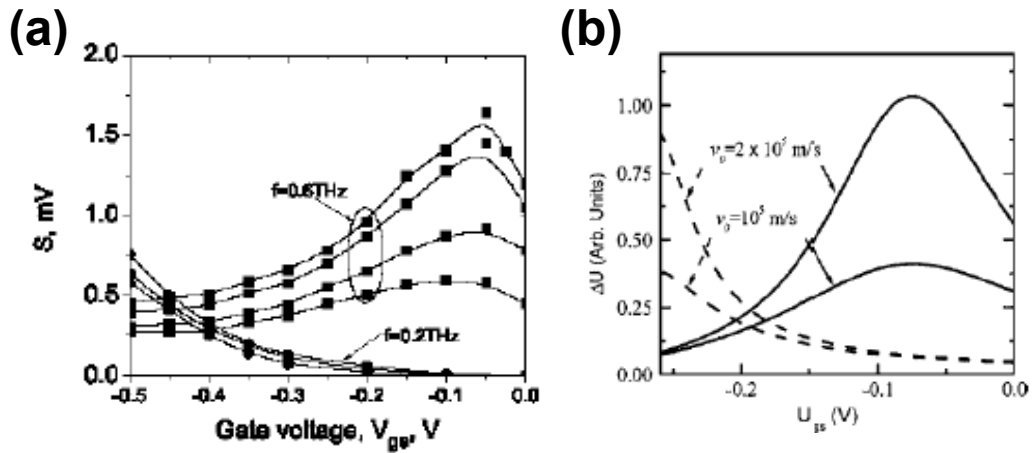
Figure 4.5 : (a) Tension source-drain photo induite en fonction de la tension de grille à 200 et 600 GHz pour différentes valeurs de la tension drain-source correspondant au courant appliqué.(b) Calculs du signal de photoconductivité en utilisant les équations du modèle Dyakonov-Shur aux fréquences 200 GHz (lignes pointillées) et 600 GHz (lignes pleines).
