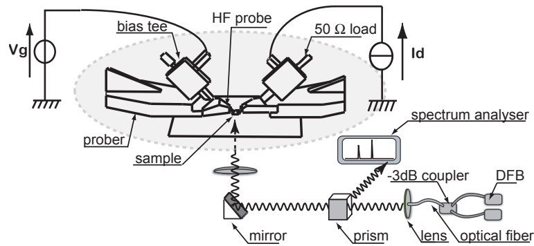
Figure 4.11 : Dispositif expérimental du battement sub-téraHertz de 2 lasers accordables émettant aux longueurs d'onde télécom.
