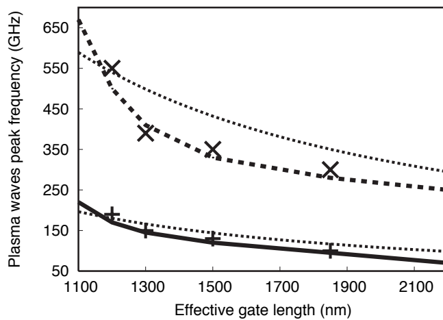
Figure 4.15 : Comparaison de la fréquence des pics d'oscillation plasma à f_0 et 3f_0 en fonction de la longueur de cavité effective obtenu expérimentalement (croix) et obtenue par le modèle hydrodynamique (points et lignes pointillées).
