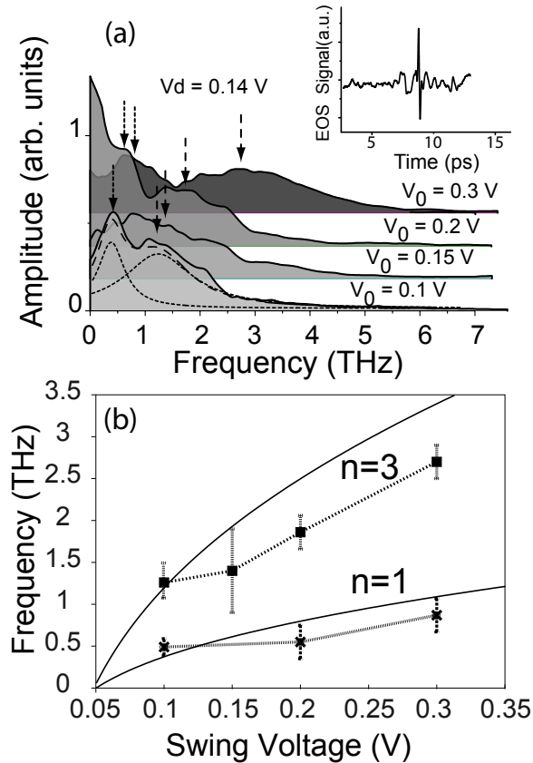
Figure 4.27 : (a) Variation des spectres d'émission mesurés par REOS en fonction de la tension de swing prise entre 0.1 V et 0.3 V. Insert : Réponse temporelle. Les lignes en pointillés et en traits discontinus sont des "fits" par une fonction de Lorentz de la courbe à V_0 = 0.1 V (b) Dépendance en fréquence des pics en fonction de la tension de swing. Les lignes en traits continus ont été calculées par l'équation (4.25) avec n=1 et n=3 .
