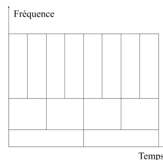
Pavage du plan temps / fréquence de la transformée en ondelettes.
