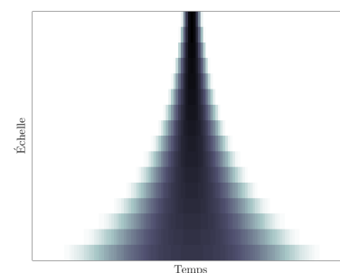
FIGURE 13: Scalogramme d'une impulsion de Dirac.
