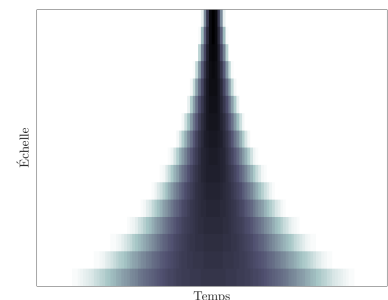
FIGURE 13: Scalogramme d'une impulsion de Dirac.
