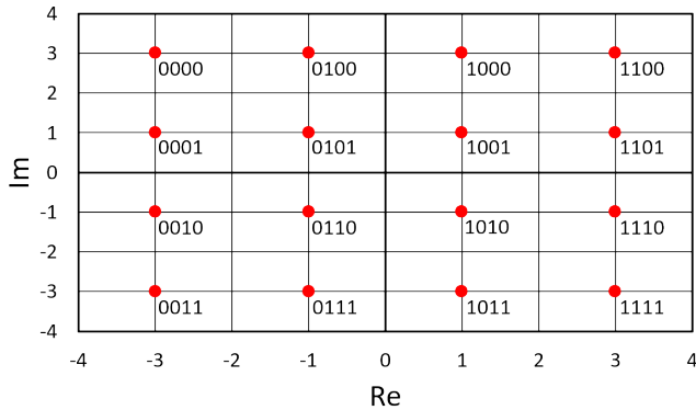
Figure 5.3 – Exemple de définition d'un alphabet OFDM sur un repère complexe (constellation 16-QAM)
