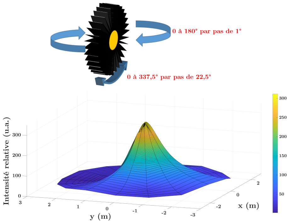
Figure 8.13 – Homogénéité radiale de la LED fort éclairement
