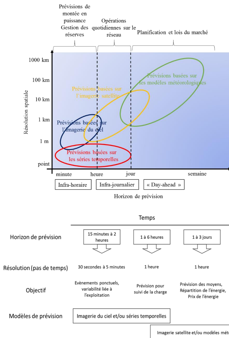
Figure III-1: En haut la résolution temporelle et horizon pour les différentes méthodes de prévision. En bas les relations entre l'horizon de prévision, les différents modèles et les objectifs (Diagne et al. , 2013)
