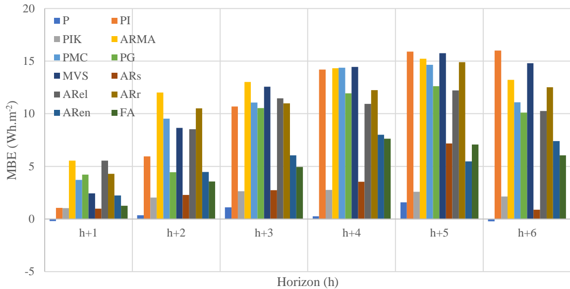
Figure IV-10: MBE en fonction de l'horizon pour les prévisions sur les données de Nancy
