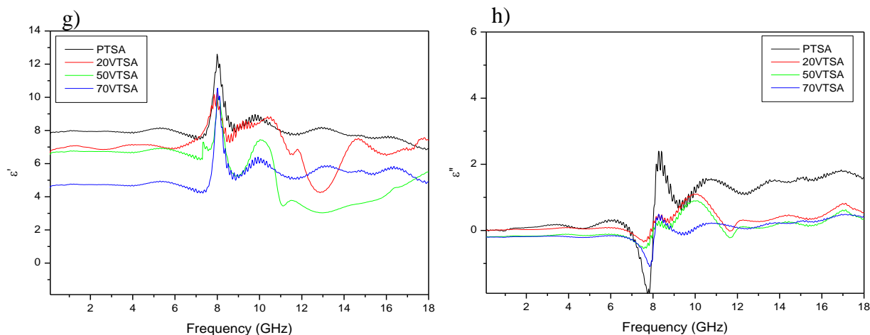
Figure V. 12. Évolution des spectres de permittivité réelle et imaginaire des composites Polyaniiline/ \text{BaFe}_{12}\text{O}_{19} synthétisés en présence de HCl (a et b) ; CSA (c et d) ; NSA (e et f) et TSA (g et h)
