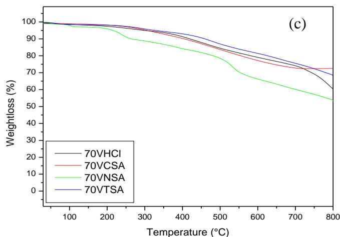
Figure IV. 28. Courbes TG des échantillons synthétisés en présence des différents acides a) Polyaniline ; Pani/BaFe 12 O 19 avec b) 20 % et c) 70 % en ferrite
