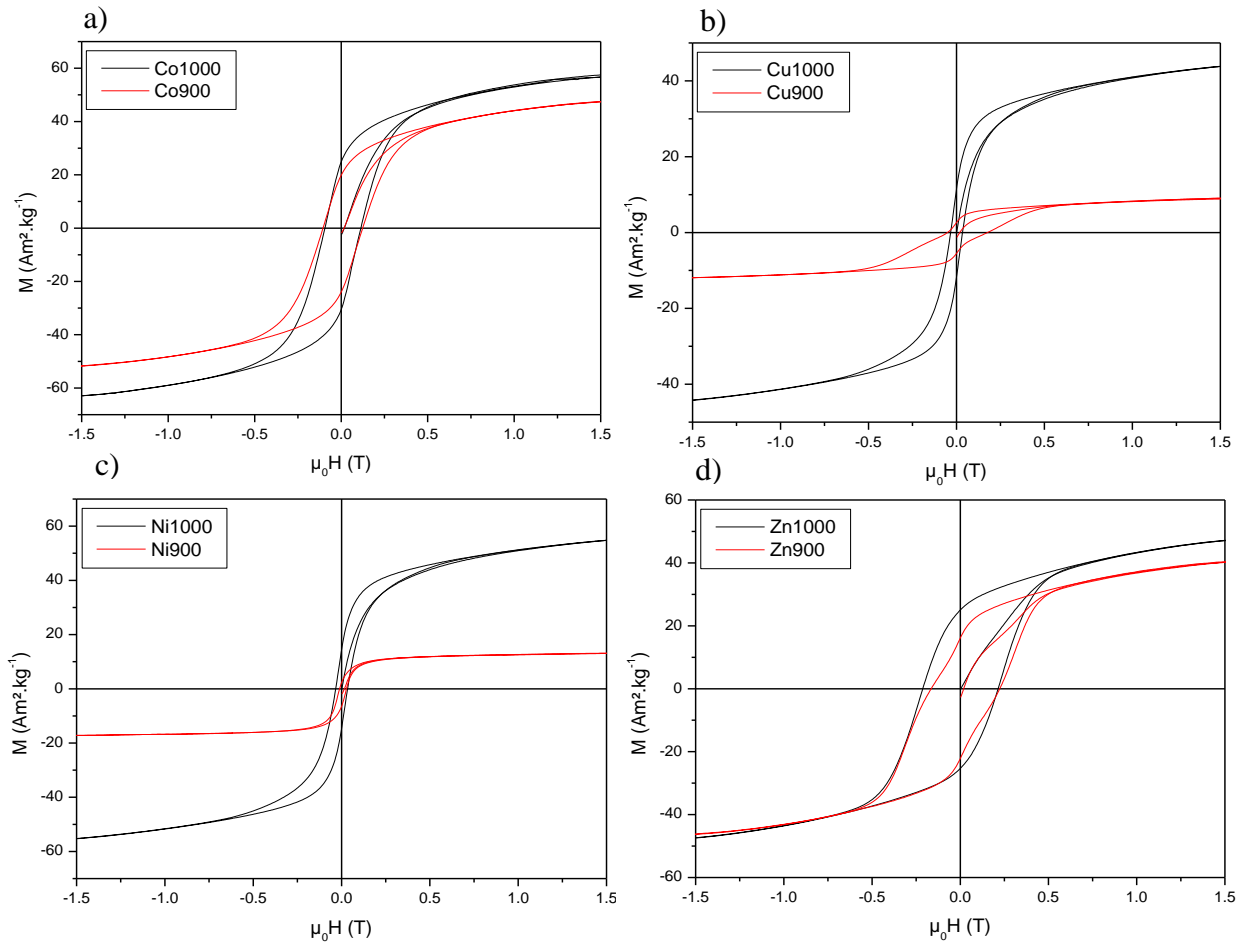
Figure III. 22. Cycles hystérésis ( M-H ) de a) \text{BaCoFe}_{11}\text{O}_{19} , b) \text{BaCuFe}_{11}\text{O}_{19} , c) \text{BaNiFe}_{11}\text{O}_{19} , c) \text{BaZnFe}_{11}\text{O}_{19} et d) \text{BaZrFe}_{11}\text{O}_{19} calcinés à différentes températures
