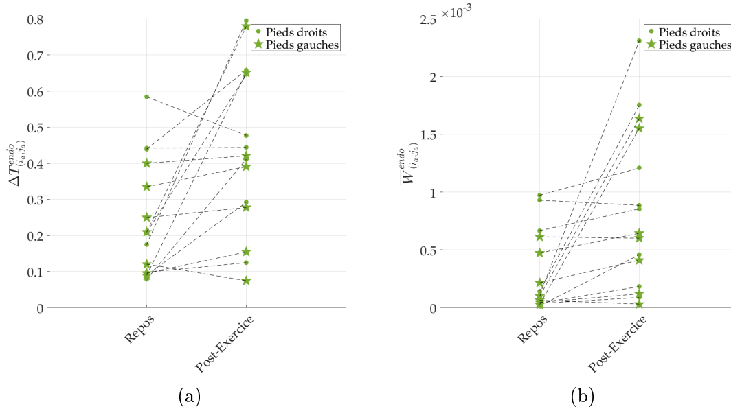
FIGURE 4.3 – Exemple d'extraction de paramètre. (a) Amplitude maximale du signal extrait de la zone active ( \Delta T_{(i_a,j_a)}^{endo} ), filtré dans la bande endothéliale. (b) Coefficient moyen d'ondelette du même signal ( \bar{W}_{(i_a,j_a)}^{endo} ).
