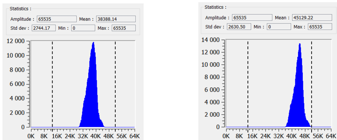
FIGURE 3.5 – Histogramme du signal pour (à gauche) un corps noir à 20 °C et (à droite) un corps noir à 40 °C. Les réglages correspondants sont les suivants : TI = 61.4 \mu s et un facteur multiplicateur de 2.6. L'axe des abscisses correspond au NI reçu par les capteurs et l'axe des ordonnées correspond au nombre de capteurs. Les traits pointillés représentent 20% et 80% du niveau maximum.
