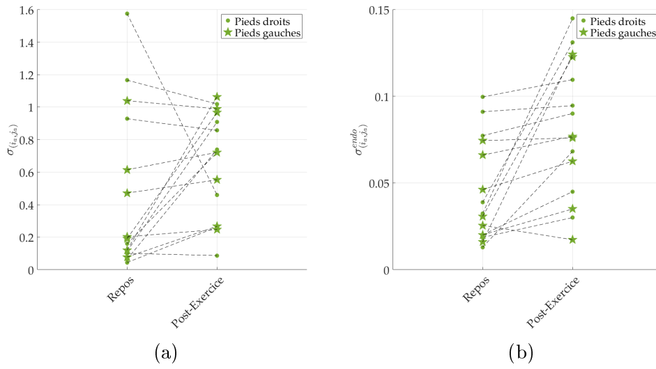
FIGURE 4.31 – Exemple d'extraction de paramètre. (a) Ecart type du signal brut extrait de la zone active \sigma_{(i_a, j_a)} . (b) Ecart type du même signal, filtré dans la bande endothéliale \sigma_{(i_a, j_a)}^{endo}
