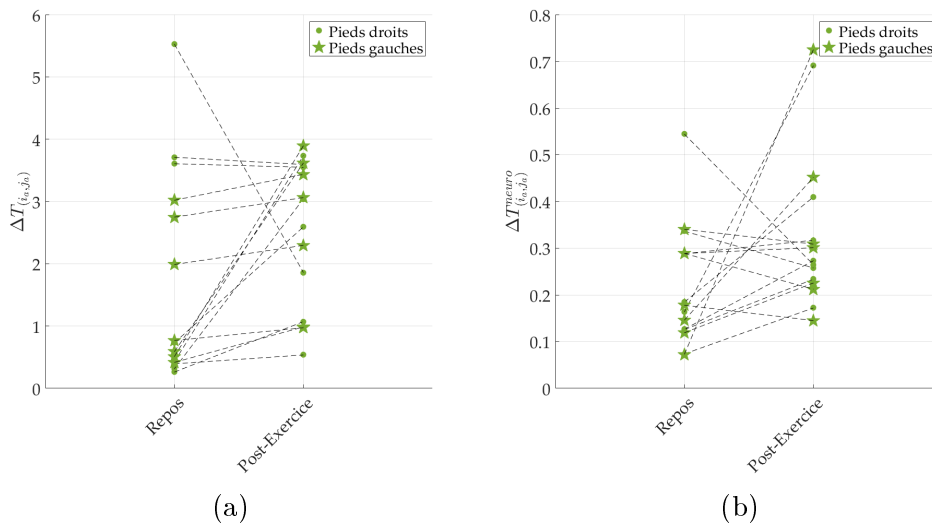
FIGURE 4.30 – Exemple d’extraction de paramètre. (a) Amplitude maximale du signal brut extrait de la zone active \Delta T_{(i_a,j_a)} . (b) Amplitude maximal du même signal, filtré dans la bande neurogénique \Delta T_{(i_a,j_a)}^{neuro} .
