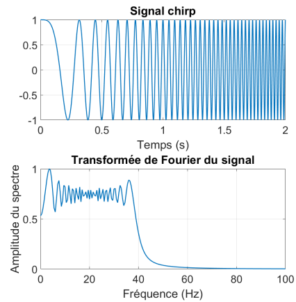
FIGURE 3.16 – Signal modulé en fréquence et sa transformée de Fourier associée.
