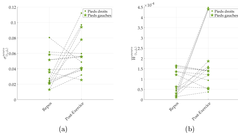
FIGURE 4.32 – Exemple d'extraction de paramètre. (a) Écart type du signal extrait de la zone active, filtré dans la bande neurogénique \sigma_{(i_a, j_a)}^{neuro} . (b) Coefficient moyen d'ondelette du même signal \overline{W}_{(i_a, j_a)}^{neuro} .
