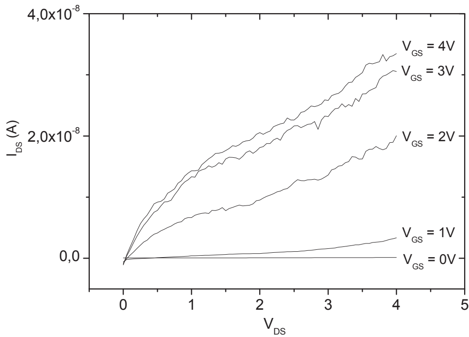
Figure 67 : caractéristiques de sortie I_{DS}(V_{DS}) pour un TFT à base de nanofils de silicium : rayon de courbure de W = 100 \text{ nm} , L=10 \text{ }\mu\text{m}
