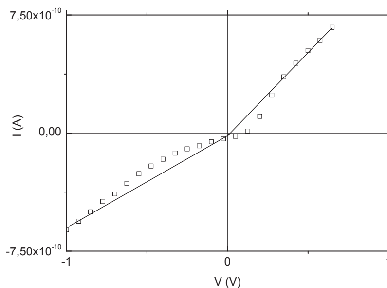
Figure 76 : courbe I-V pour des nanofils de 50nm de hauteur – 8 \mu m de longueur
