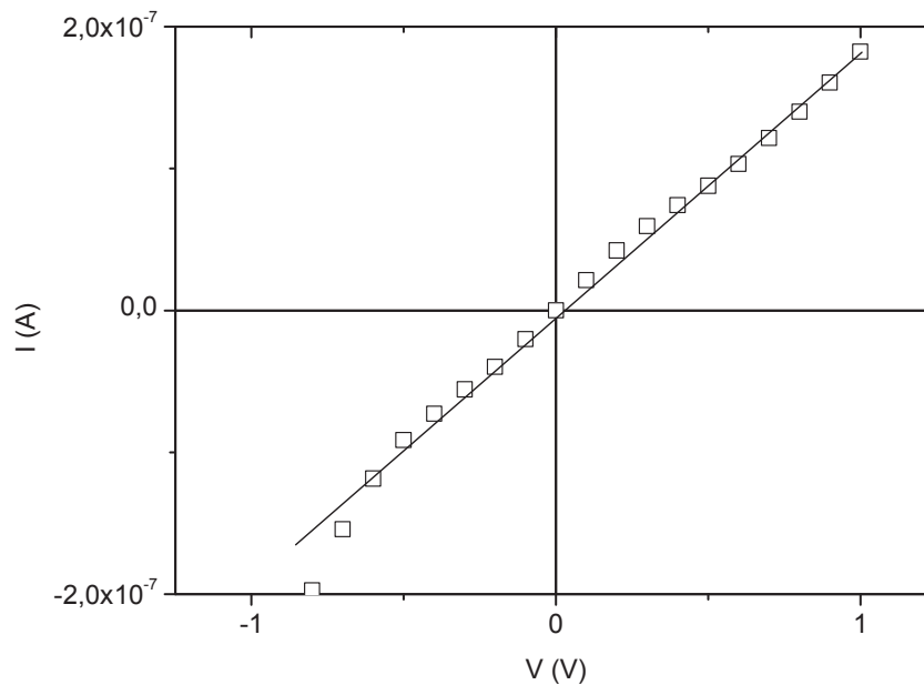
Figure 77 : courbe I-V pour des nanofils de 200nm de hauteur -- 8 \mu m de longueur
