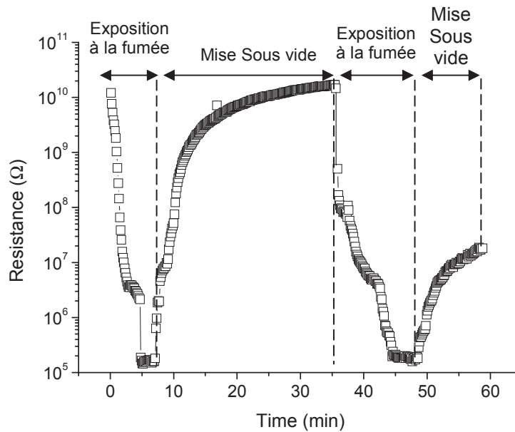
Figure 80 : évolution de la résistance électrique en fonction du temps : effet de la fumée. Rayon de courbure des nanofils 100nm.
