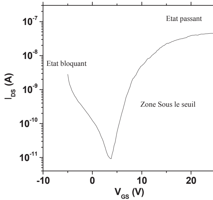
Figure 66 : caractéristique de transfert I_{DS}(V_{GS}) pour un TFT à base de nanofils de silicium : rayon de courbure de W = 100 \text{ nm} , L = 10 \text{ }\mu\text{m} , V_{DS}=4\text{V}
