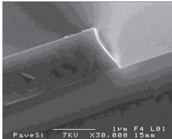
Figure 28 : cliché MEB d'une vue en coupe d'une marche de silicium polycristallin obtenue après gravure sèche dans les conditions standards du laboratoire : pression 30mT, puissance 30W, débit de SF 6 = 20sccm
