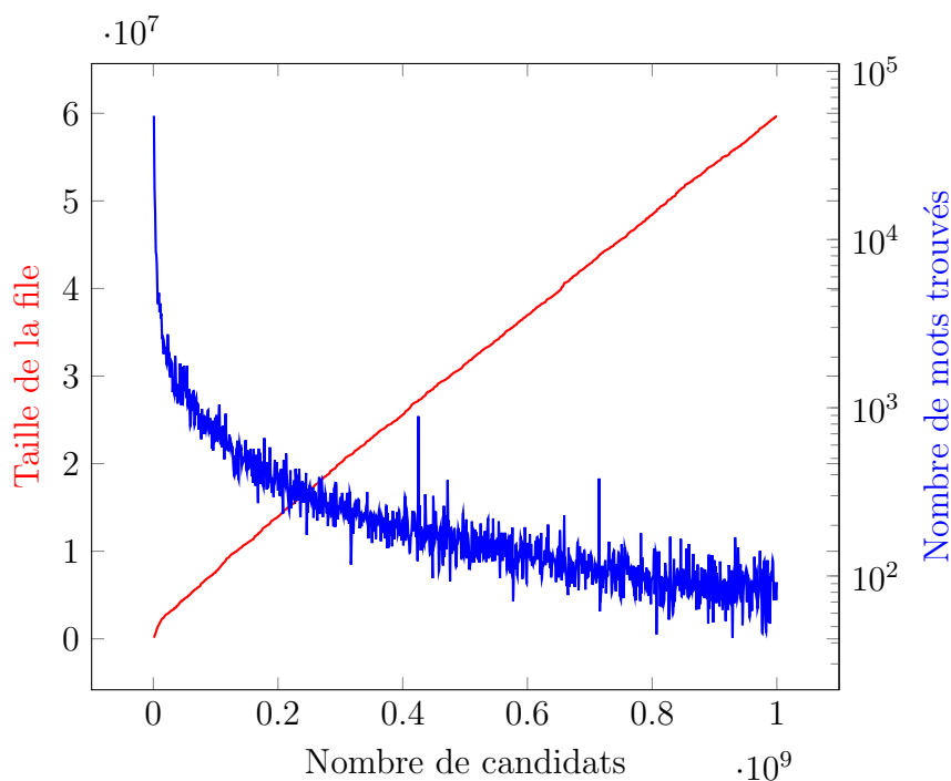
FIGURE 6.7 – Rockyou avec seuil = 10^4
