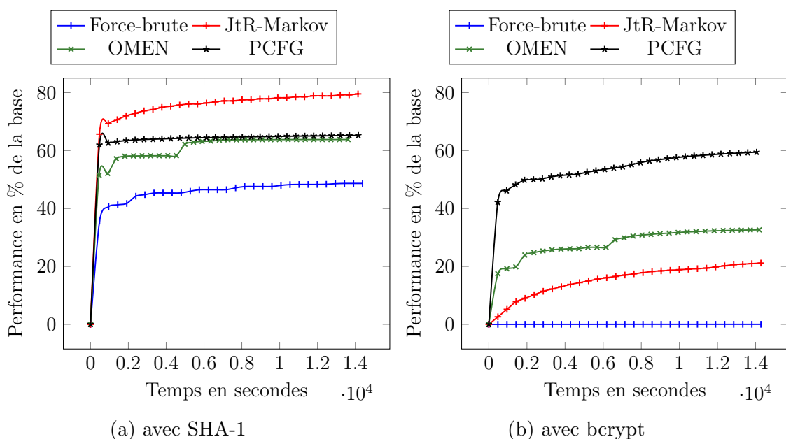
FIGURE 4.6 – Attaque sur Rockyou
