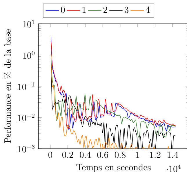
FIGURE 5.11 – Attaque de PCFG sur Rockyou avec ZXCVCBN
