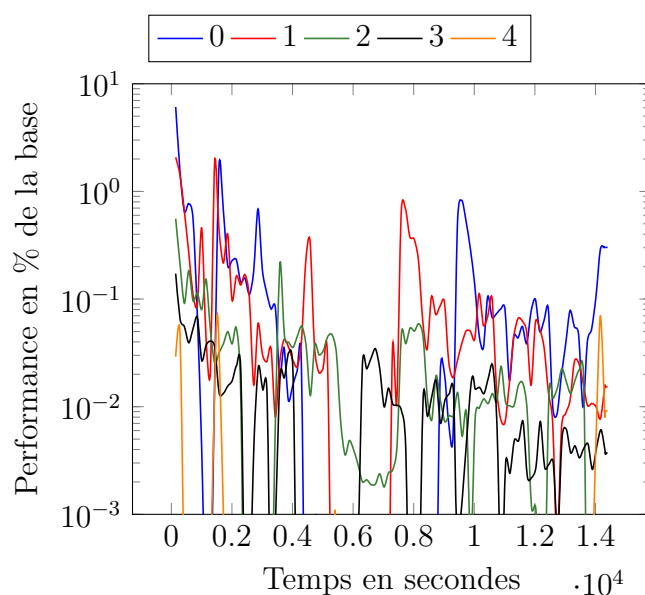
FIGURE 5.10 – Attaque de JtR-Markov sur LinkedIn avec ZXCVCBN
