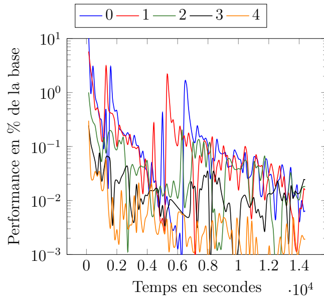
FIGURE 5.8 – Attaque de JtR-Markov sur RockyYou avec ZXCvbn
