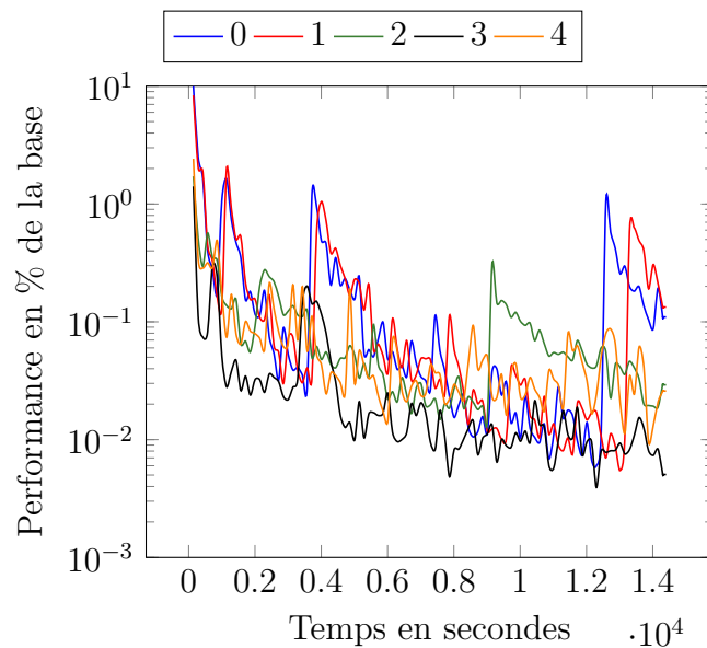
FIGURE 5.9 – Attaque de JtR-Markov sur Myspace avec ZXCvbn
