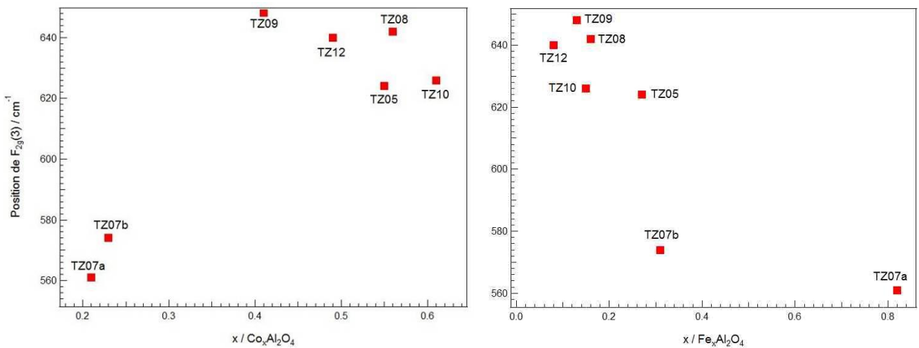
Figure II.12: Diagrammes montrant les fréquences de F_{2g}(3) en \text{cm}^{-1} versus le taux calculé de Co ou Fe dans les formules \text{CoAl}_2\text{O}_4 (gauche) et \text{FeAl}_2\text{O}_4 (droite).
