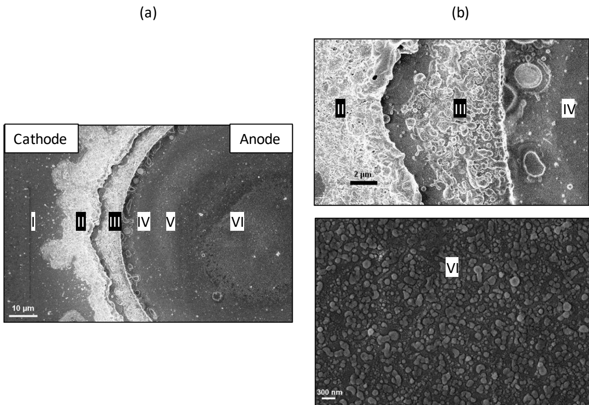
Figure 4.18. (a) Imagerie électronique en vue de dessus d'un micro réacteur planaire après utilisation en polarité inverse dans l'argon. (b) Zoom sur les zones II, III, IV et VI. Conditions expérimentales : micro réacteur avec anode en silicium, 100 µm de diamètre, argon, pression variable, 10 minutes de fonctionnement à 0,5 mA.
