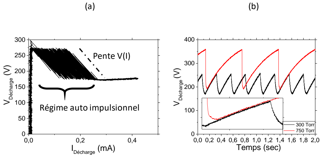
Figure 4.23. (a) Courbe V-I de la décharge dans l'argon à 500 Torr pour un courant injecté maximal de 400 \mu\text{A} et une résistance de ballast de 1 M \Omega . (b) Courbes de la tension de décharge en fonction du temps dans le régime auto impulsif pour un micro réacteur fonctionnant dans l'argon à différentes pressions avec une résistance de ballast de 1 M \Omega . Conditions expérimentales : diamètre 100 \mu\text{m} , profondeur 55 \mu\text{m} .
