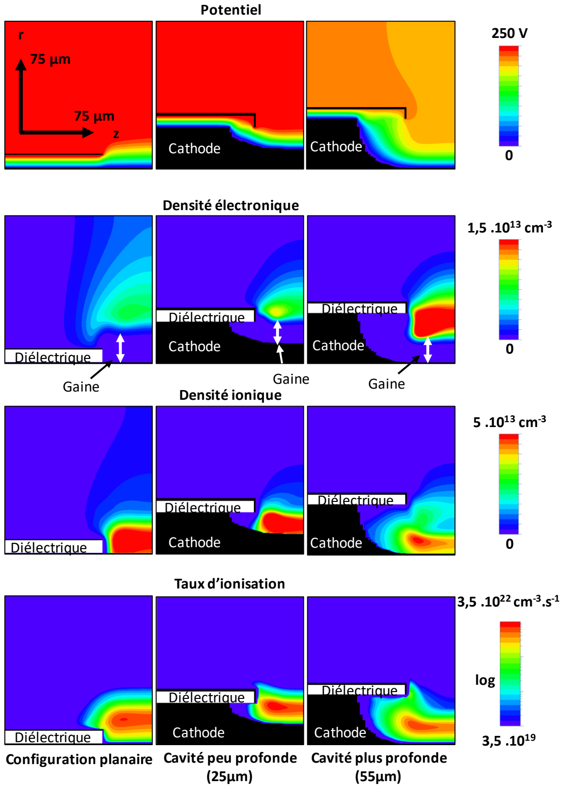
Figure 4.34. Simulation du potentiel, des densités électronique et ionique et du taux d'ionisation pour une microdécharge en polarité directe dans l'hélium à 800 Torr de 100 μm de diamètre pour différentes géométries.
