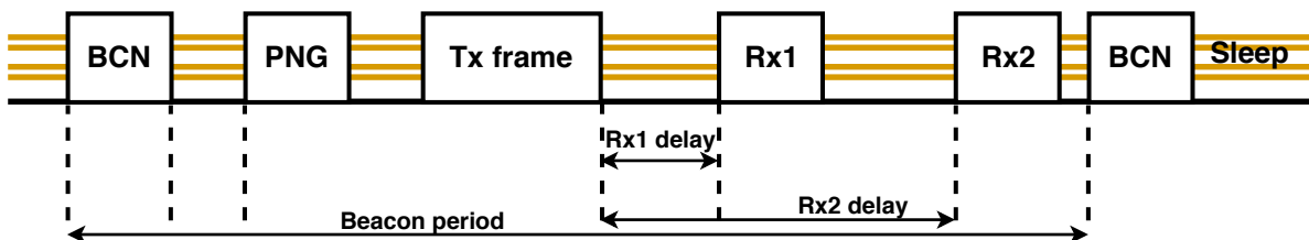
FIGURE 2.5 – Fenêtres de la Classe B.
