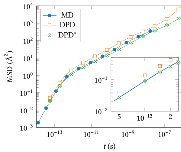
FIGURE 3.30 – Utilisation d’un modèle DPD avec masse effective. La masse des grains du modèle DPD* est calculée d’après l’équation (3.39), de sorte que le MSD des grains à 2 \Delta t = 10^{-13} s coïncide avec la référence MD. Le MSD calculé avec le modèle DPD* est meilleur qu’avec le modèle DPD classique.
