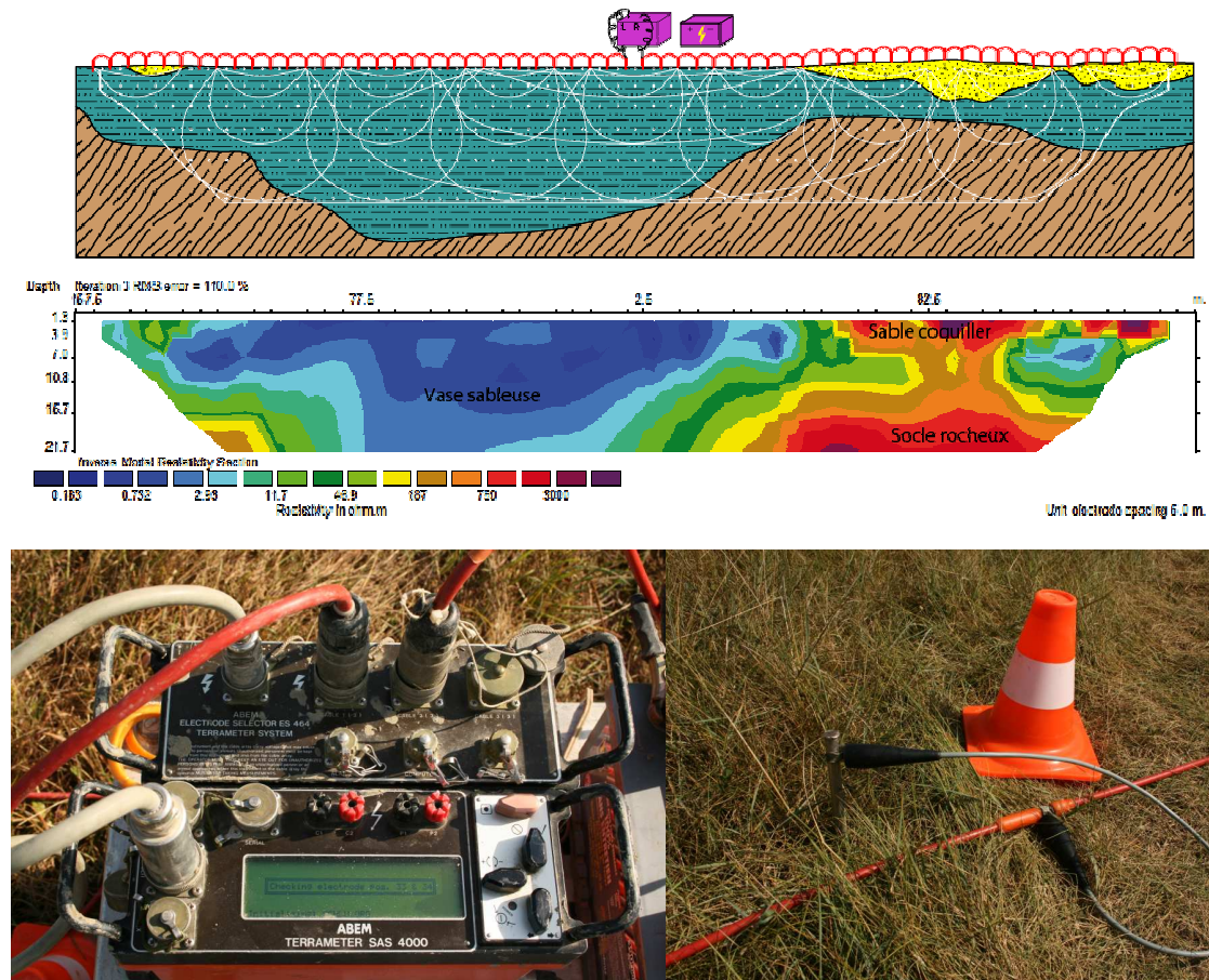
Figure II.3 : Dispositif de mesure de tomographie électrique.
