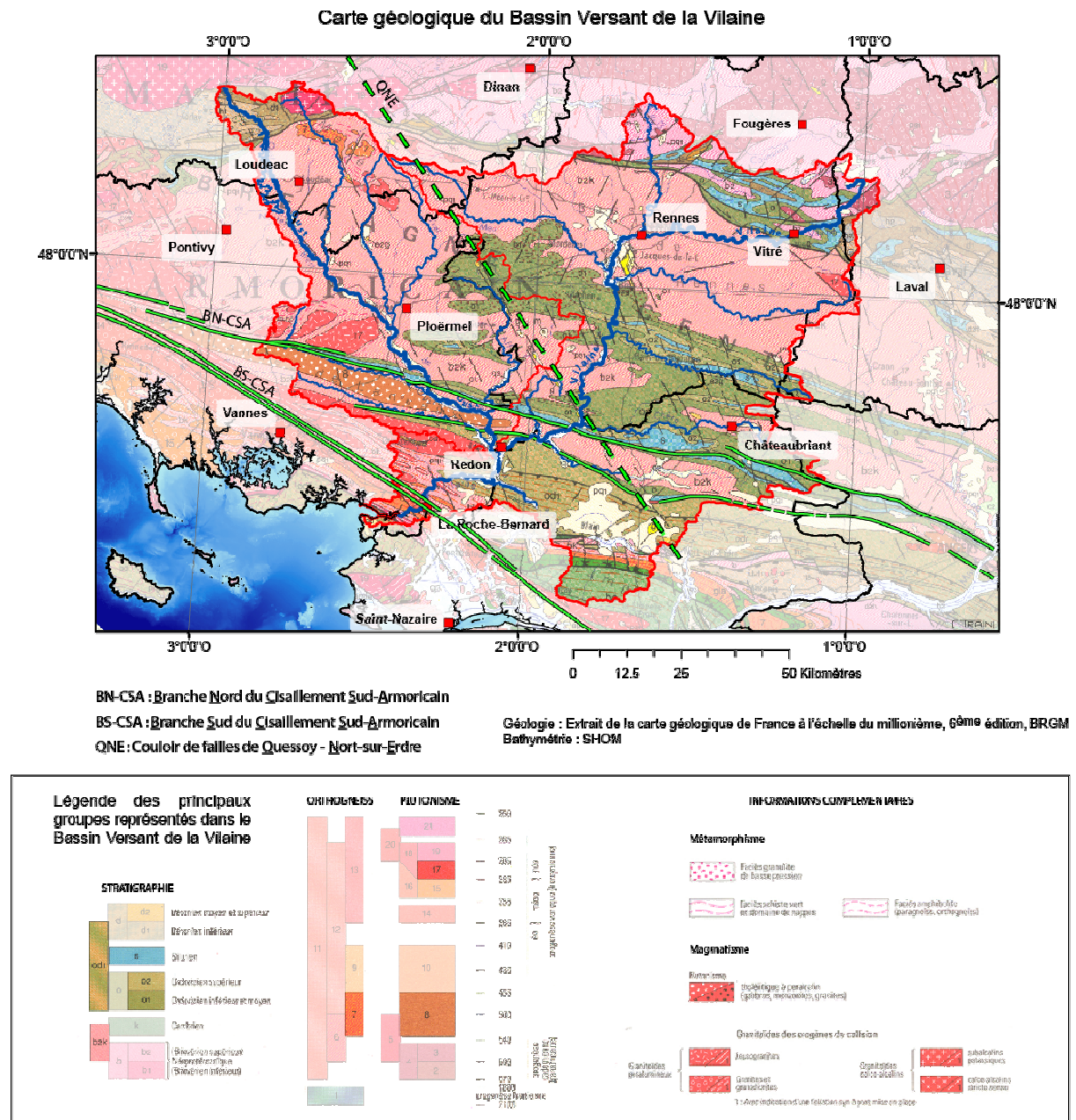
Figure I.4 : Carte géologique du bassin versant de la Vilaine.
