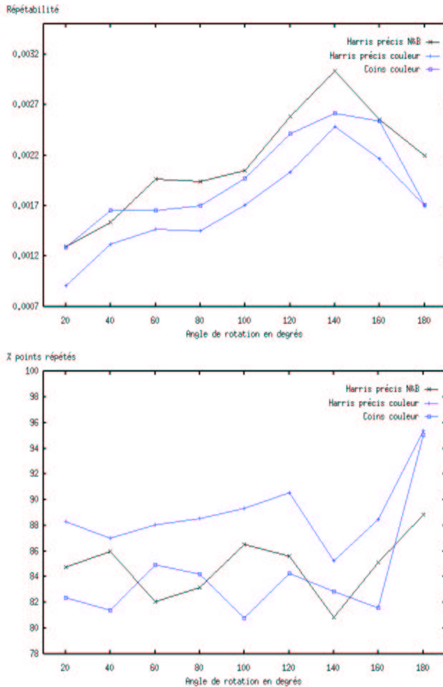
Figure 2.6 – Séquence “Salle robotique” : Répétabilité R^1 suivant 9 rotations image.
