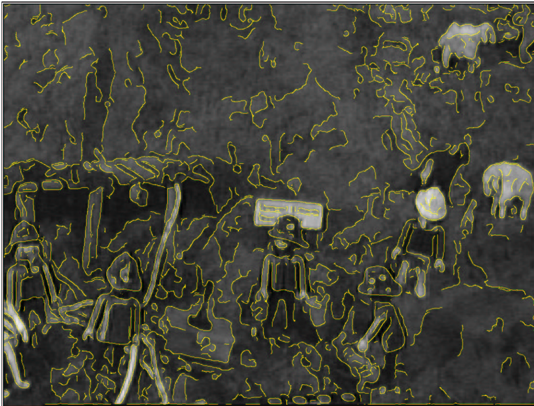
Figure D.14 – Détection de contours couleur en précision sub-pixel par la méthode MAX : détail des “personnages”.
