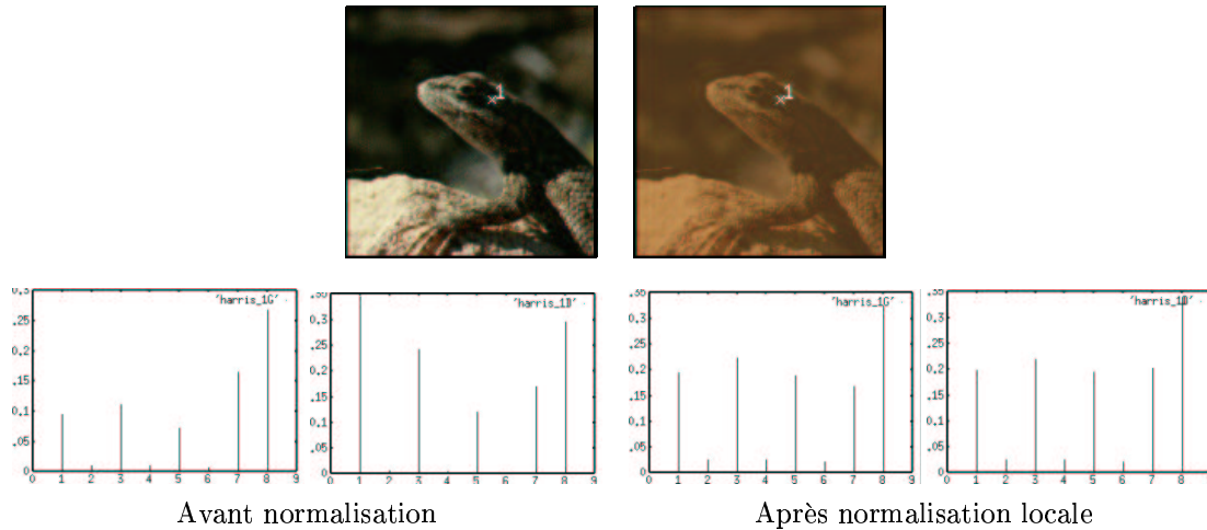
Figure 4.6 – Les deux vecteurs d'invariants couleurs obtenus avant et après normalisation.
