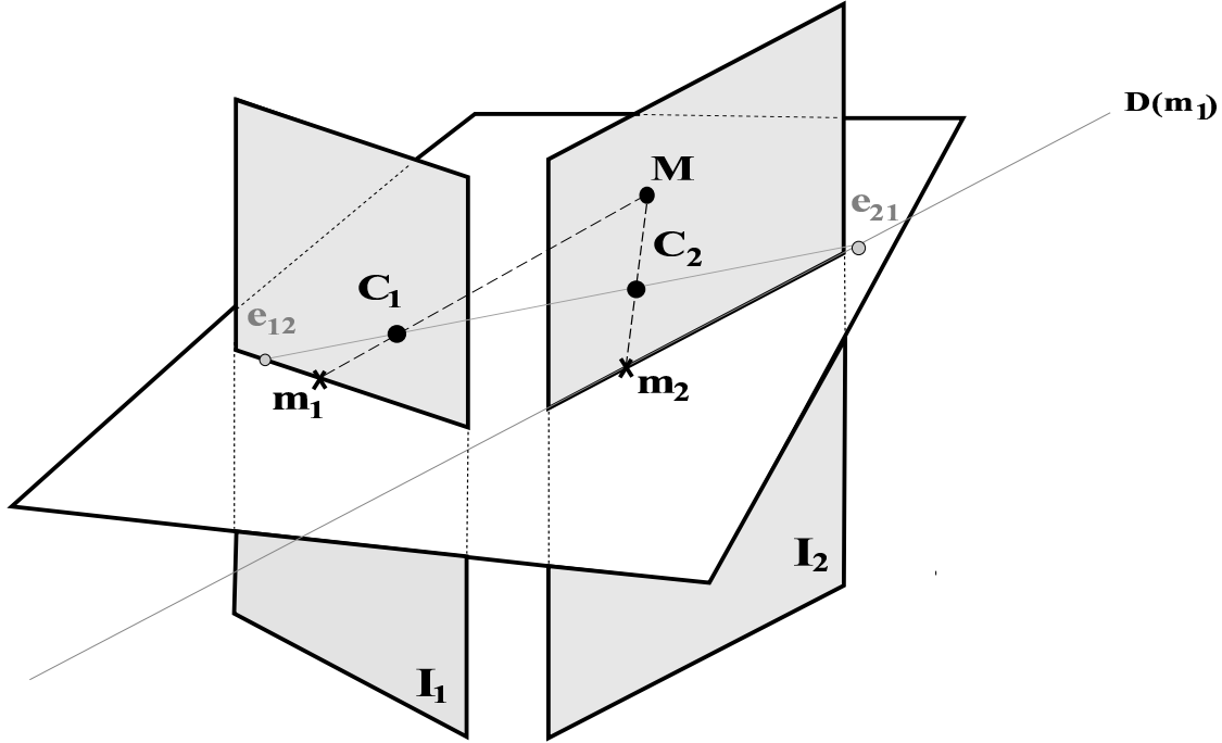
Figure 7.4 – Géométrie épipolaire d'un système de deux caméras.
