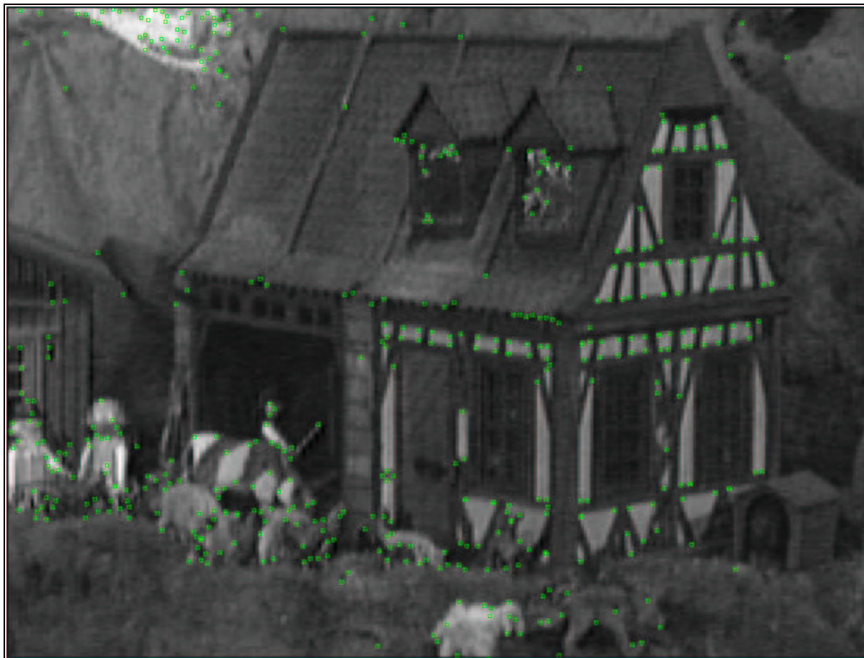
Figure D.17 – Détection de coins couleur en précision quart de pixel (détail des “maisons”).
