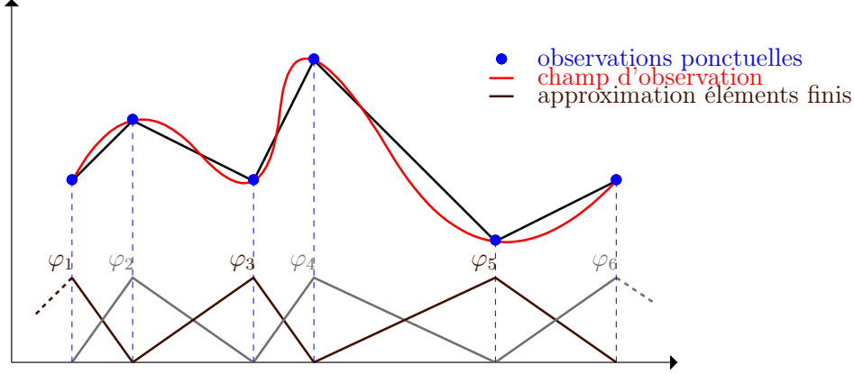
FIGURE 1.8 – Lien entre le champ d’observation (en rouge), sa représentation en éléments finis (en noir) et les observations ponctuelles (en bleu). Sont représentées en bas les fonctions de pondération ( \varphi_l ) associées aux données ( y_l ).
