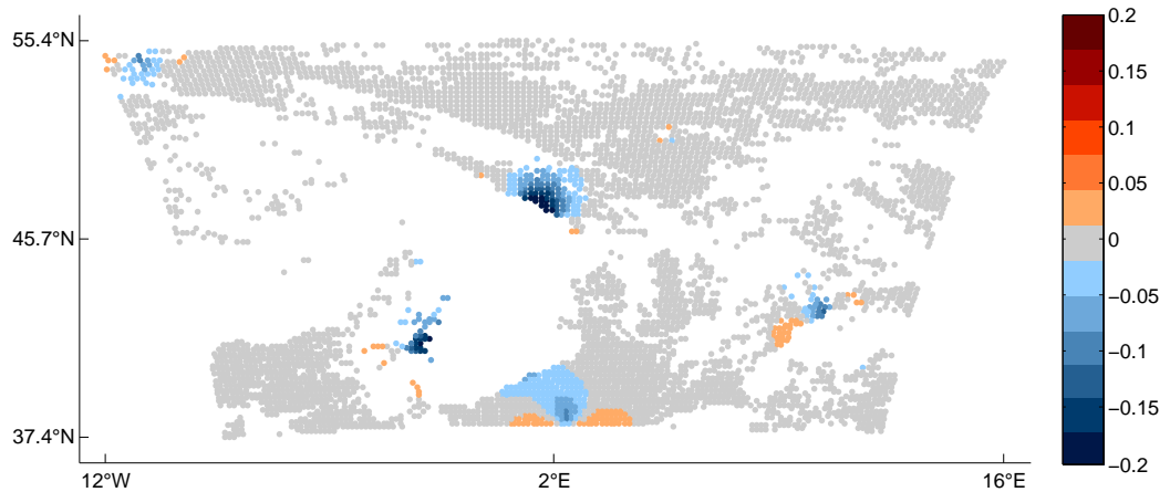
FIGURE 4.20 — Écarts à la solution analytique correspondant aux expériences de la figure 4.19.
