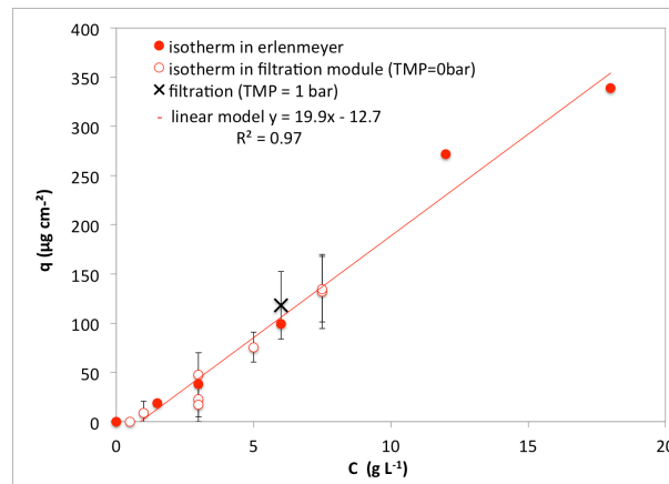
Figure 3.10 – Isotherme d’adsorption de Glutathione sur la membrane PES (KOCH, MFK-618) en Erlenmeyer (disques pleins rouges), en module de filtration sans pression (cercles rouges vides), et biomolécule accumulée sur la membrane pendant la filtration (croix noire). [HABIBI 2013]
