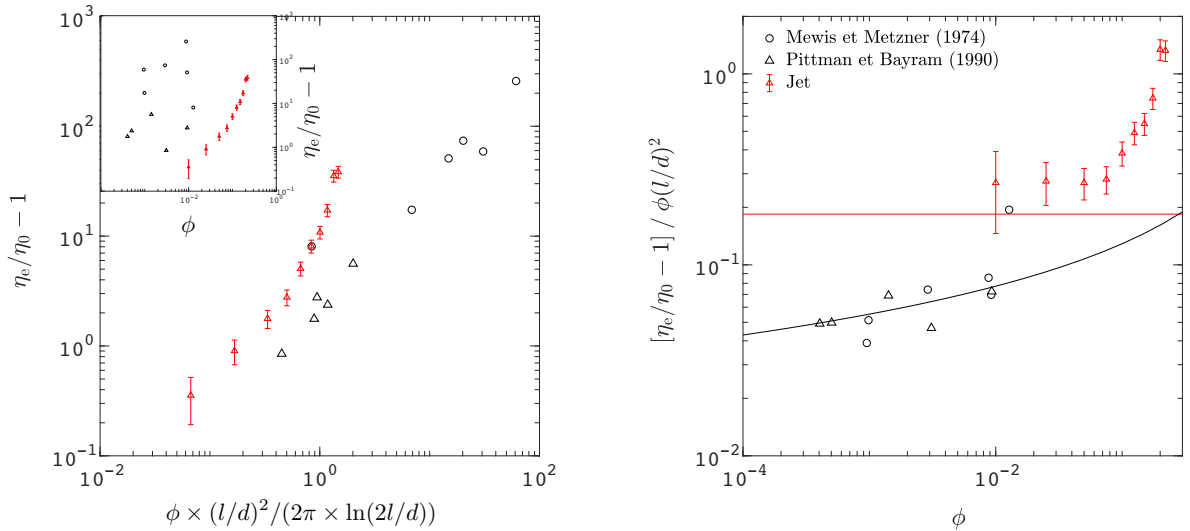
FIGURE 4.13 – a) Écart relatif à la viscosité d'un liquide newtonien en fonction de l^2/2\pi d^2 \ln(2l/d)\phi , où l^2/2\pi d^2 \ln(2l/d)\phi = 1 délimite les régimes dilué et concentré. Les données tracées rassemblent les mesures présentées précédemment ainsi que des données tirées de Mewis et Metzner [63] et de Pittman et Bayram [75]. L'insert représente l'écart relatif à la viscosité d'un liquide newtonien en fonction de \phi . b) Valeur de (\eta_e/\eta_0 - 1) compensée de \phi(l/d)^2 en fonction de \phi et prédictions des régimes dilué (—) et concentré (—).
