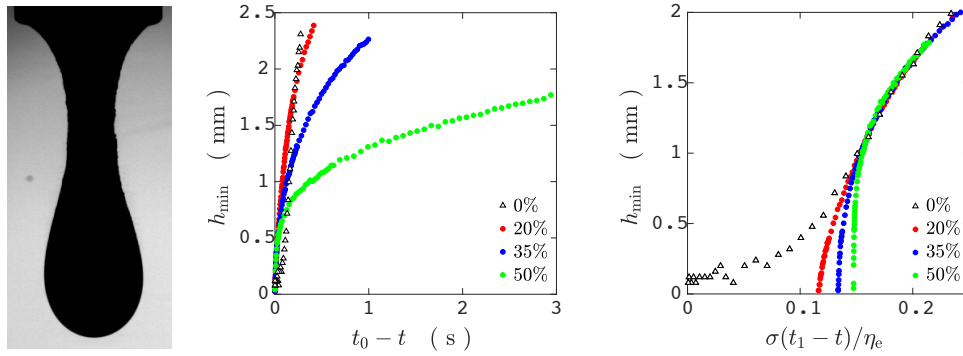
FIGURE 2.5 – Gauche : profil typique d'une goutte pendante de billes de 80 \mu\text{m} en suspension dans du PEG. Centre : évolution temporelle de h_{\min} pour des gouttes pendantes se détachant d'une buse. Les cercles pleins correspondent à des suspensions de billes de polystyrène de diamètre d = 80 \mu\text{m} suspendues à diverses fractions volumiques. Les triangles correspondent eux au liquide pur (PEG). Droite : mêmes données, ajustées et décalées par un temps arbitraire t_1 de façon à les superposer lors des premiers instants du pincement au cas de référence du liquide pur ( \phi_0 )
