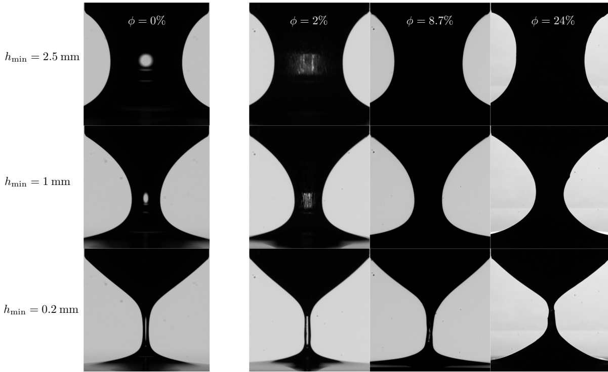
FIGURE 4.3 – Pincement de ponts capillaires illustré pour des diamètres minimaux h_{\min} = 2.5, 1 et 0.2 mm. La séquence de gauche montre un liquide newtonien de viscosité ( \eta_0 = 2.88 Pa \cdot s). Celle de droite montre une suspension de fibres à des fraction volumique \phi = 2\% , 8.7\% et 24\% dans un liquide newtonien (de viscosité \eta_0 = 2.88 Pa \cdot s pour les deux premières et \eta_0 = 0.25 Pa \cdot s pour la dernière). Toutes les dynamiques sont limitées par la viscosité ( Oh \gtrsim 1 ). L'image encadrée en rouge est une visualisation permettant de mettre en évidence l'aligement des fibres au sein de l'écoulement ( \phi = 1\% ).
