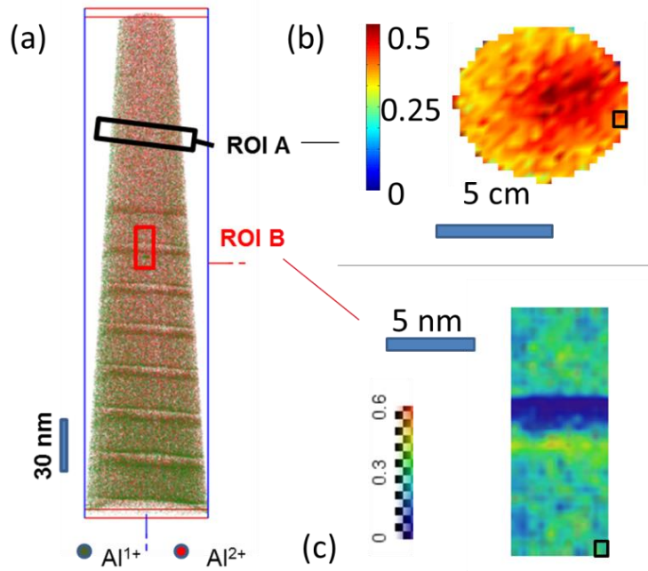
Fig. 2.6. Un volume reconstruit après une analyse de SAT peut être filtré spatialement pour en extraire des sous-volumes, tels les régions d'intérêt (ROI) A et B (a). En (b), la fraction de site d'Al dans l'AlGaIn (voir section 4.2) est exprimée dans l'espace du détecteur pour la ROI A. En (c), la même quantité est calculée dans l'espace reconstruit pour la ROI B (on visualise une coupe 2D d'un volume 3D). Le carré noir indique respectivement la taille du pixel et du voxel.
