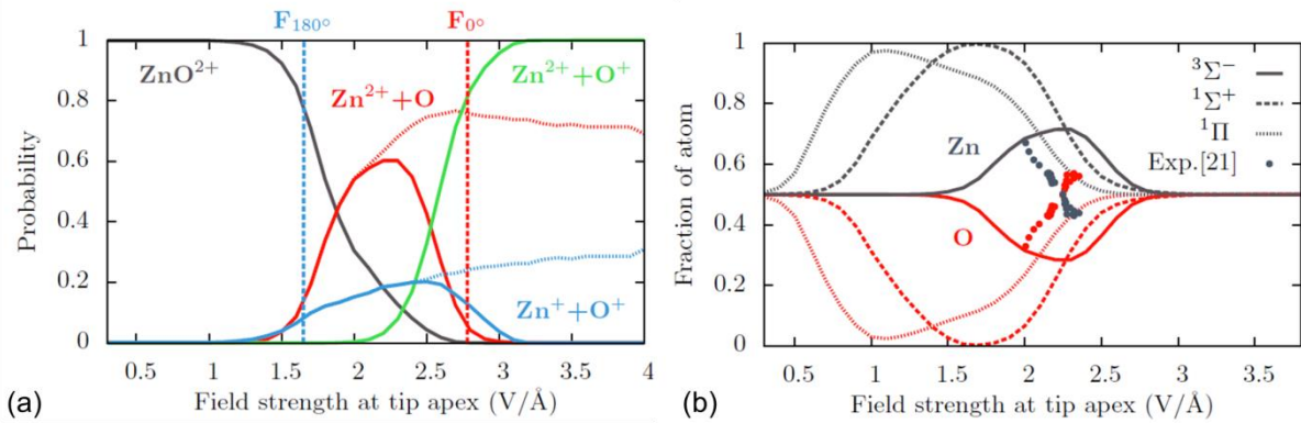
Fig. 3.10. (a) Probabilité de trois différents canaux de sortie d'une molécule de ZnO^{2+} en fonction du champ électrique à la surface d'une pointe d'émission de champ. La molécule est supposée s'évaporer dans l'état 1^3\Sigma^- . Les courbes hachées correspondent à la simple réaction de dissociation ZnO^{2+} \rightarrow Zn^{2+}+O et ZnO^{2+} \rightarrow Zn^++O^+ , sans la post-ionisation de l'O et du Zn^+ , respectivement. Les lignes verticales indiquent les champs critiques pour la molécule mère orientée à 0^\circ (Zn devant) et à 180^\circ (O devant) avec le champ électrique. (b) Mesure de la fraction atomique en SAT conséquente aux réactions de dissociation/post-ionisation de la molécule de ZnO^{2+} . Les trois courbes correspondent à des différents états de départ pour la molécule mère ZnO^{2+} .
