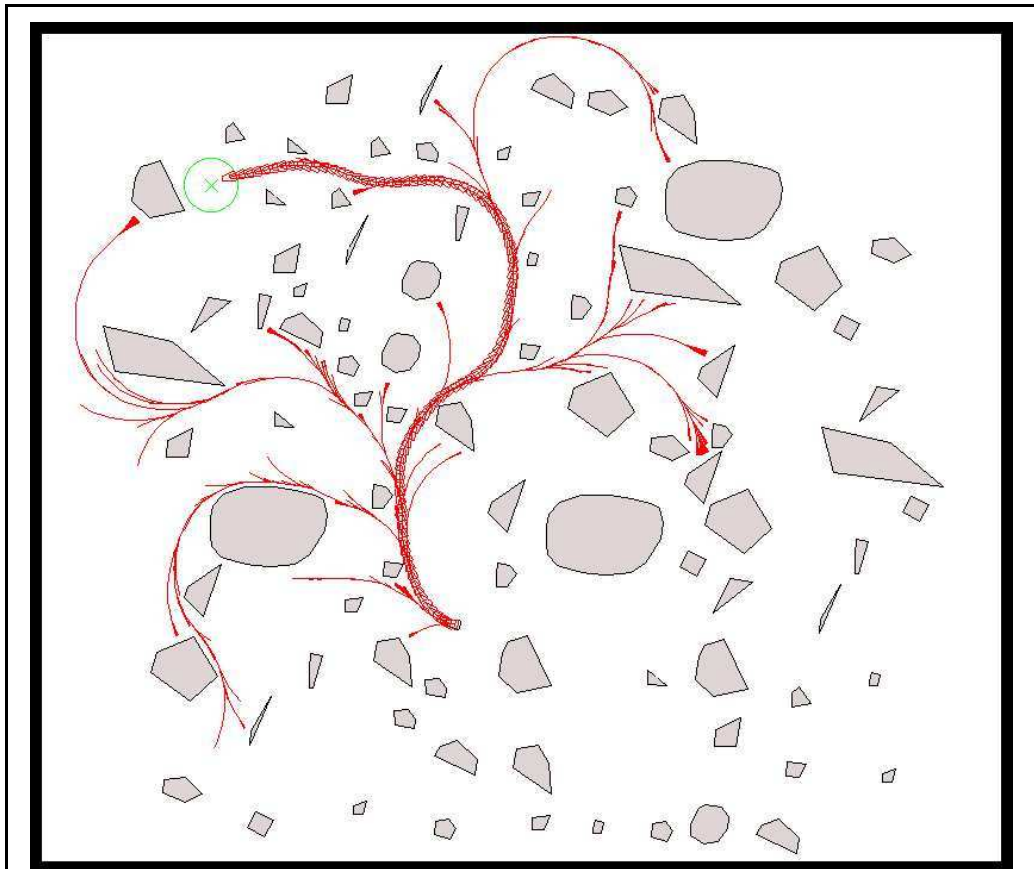
FIG. C.4 – Exemple de LR\ Gauss\ VGB_{10} dans un champ d'obstacles.
