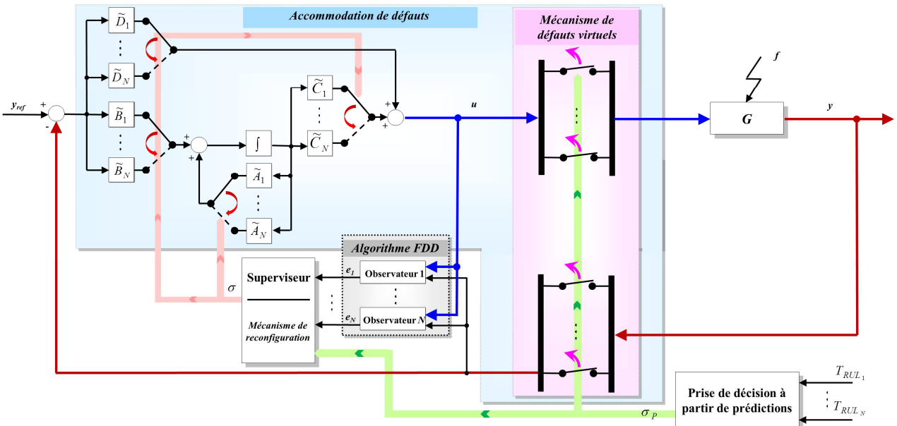
Figure 4.3 – Détails de l'architecture ADAcom
