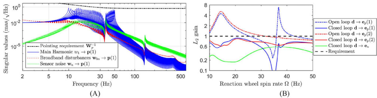
Figure 3.46 – (A) Pour différentes vitesses \Omega , contributions des perturbations sur l'erreur de pointage, (B) gains \ell_2 du transfert de d \rightarrow e vers chaque signaux objectifs pondérés
