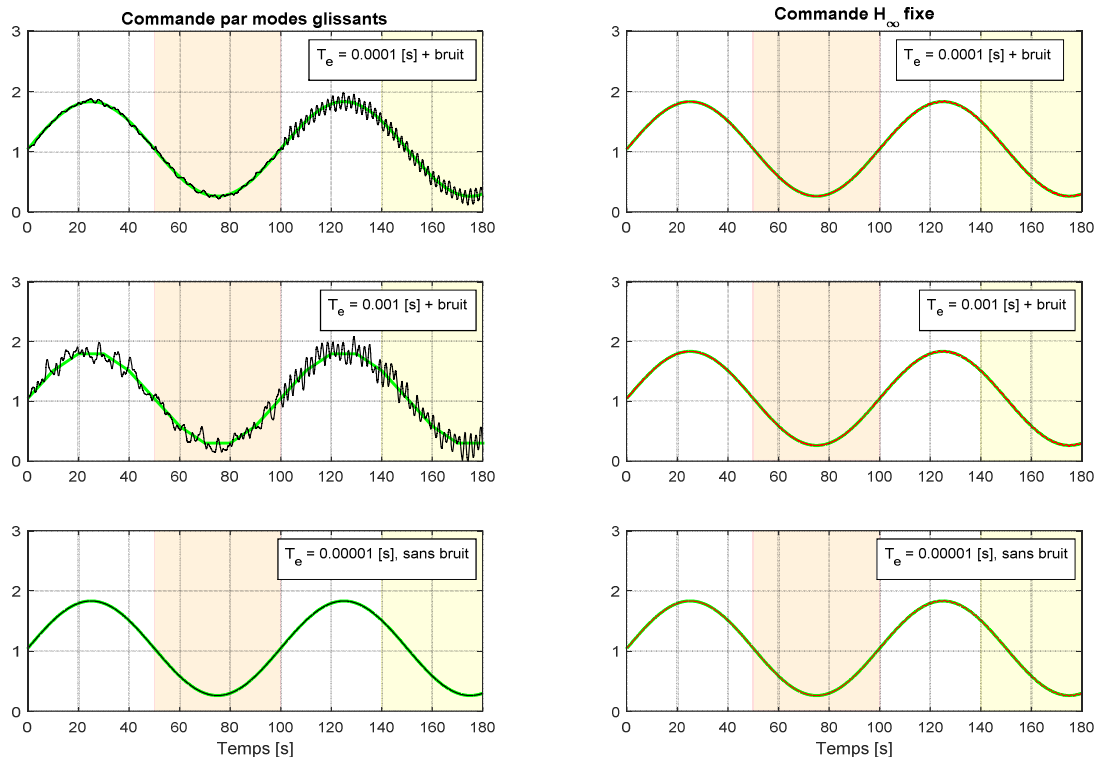
Figure 2.28 – Signal contrôlé pour différentes fréquences d'échantillonnage
