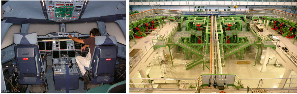
Figure 3.26 – Simulateur de vol de l’A380 et représentation Iron Bird [Gh13]
