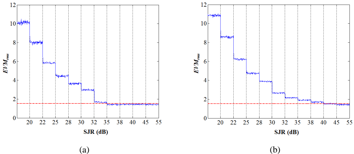
Figure 4.5. Observations de l' EVM_{rms} en fonction du SJR pour les bases de données : a : M2, b : M3.
