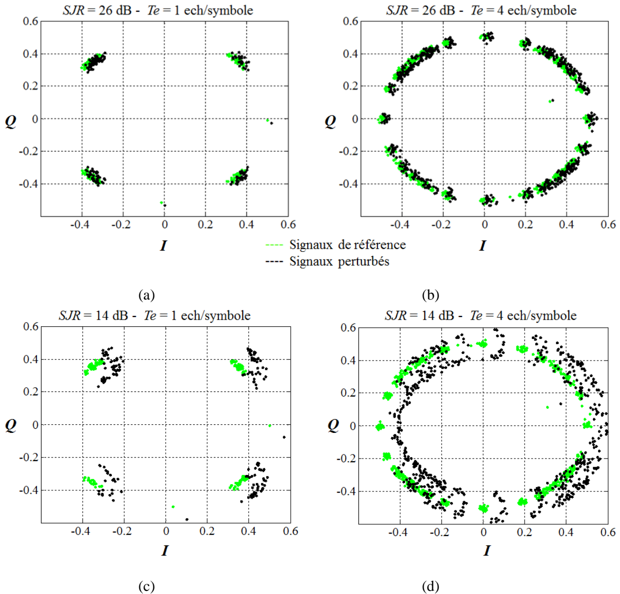
Figure 3.6. Constellations des signaux en quadrature I(nT_e) et Q(nT_e) perturbées avec G_2(t) a : SJR = 26 \text{ dB} T_e = 1 \text{ ech/symb} , b : SJR = 26 \text{ dB} T_e = 4 \text{ ech/symb} , c : SJR = 14 \text{ dB} T_e = 1 \text{ ech/symb} , d : SJR = 14 \text{ dB} T_e = 4 \text{ ech/symb} , en vert le signal de référence et en noir le signal perturbé (en simulation).
