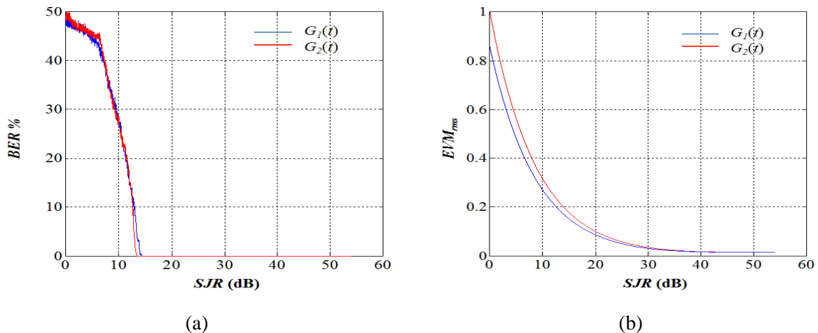
Figure 4.2. Variation du SJR avec SNR à 30 dB en présence des perturbation G_1(t) et G_2(t) pour a : le BER , b : l' EVM_{rms} (en simulation).
