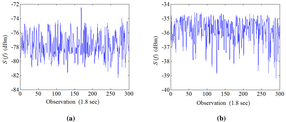
Figure 3.13. Evolutions temporelles de deux fréquences de la dsp S . observées sur banc de mesure, (a) : S(f) = 912 MHz), (b) : S(f) = 924.8 MHz) (en mesure).
