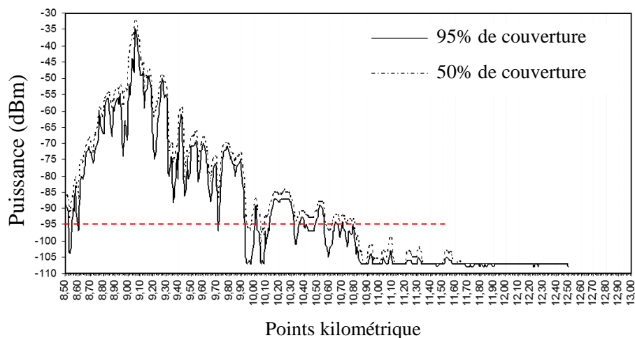
Figure 1.6. Puissance reçue sur un canal GSM-R en fonction de la distance à la BTS (source SNCF).
