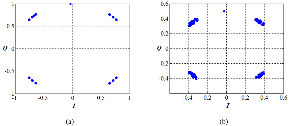
Figure 3.3. Constellations des signaux en quadrature I(nT_e) et Q(nT_e) , a : avant canal BBAG , b : après canal BBAG de SNR = 30 dB, avec un pas d'échantillonnage de 1 échantillon par symbole (en simulation).
