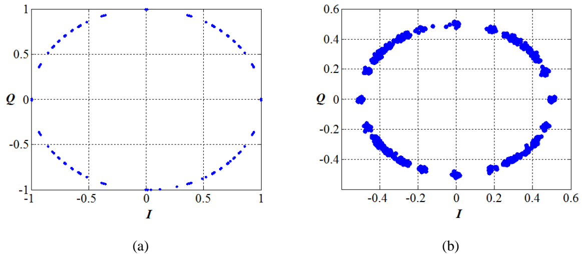
Figure 3.4. Constellations des signaux en quadrature I(nT_e) et Q(nT_e) , a : avant canal BBAG , b : après canal BBAG de SNR = 30 dB, avec un pas d'échantillonnage de 4 échantillons par symbole (en simulation).
