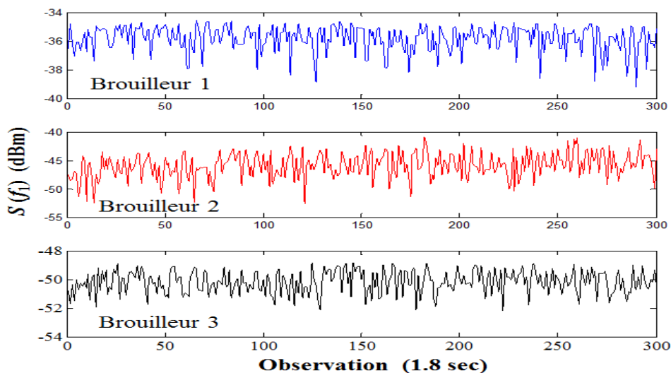
Figure 3.12. Evolution temporelle d'une fréquence observée sur banc de mesure avec f_l = 924.8 MHz pour les 3 brouilleurs (1.8 sec) (en mesure).
