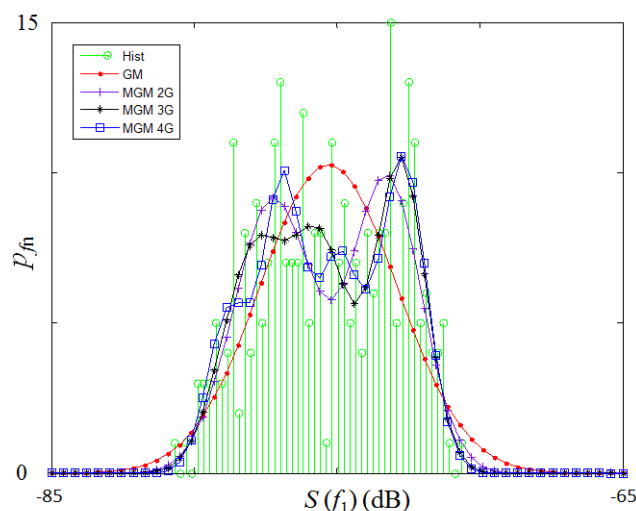
Figure 1. Histogramme et pdf de la fréquence f_1 = 924.8 MHz pour un modèle multi-gaussien G = 1, 2, 3, 4 .
