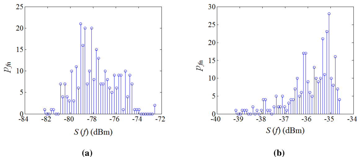
Figure 3.14. Histogrammes des 300 observations consécutives observées sur banc de mesure pour a) S(f)=912 MHz), b) S(f)=924.8 MHz) (en mesure).
