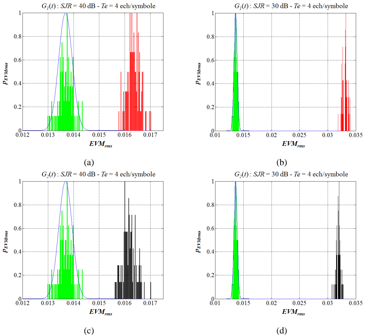
Figure 3.9. Histogrammes de l' EVM_{rms} pour le signal de référence (en vert), pour le signal perturbé G_1(t) en rouge, a : SJR = 40 \text{ dB} , b : SJR = 30 \text{ dB} , pour le signal perturbé G_2(t) en noir c : SJR = 40 \text{ dB} , d : SJR = 30 \text{ dB} , en bleu l'estimation de la distribution (en simulation).
