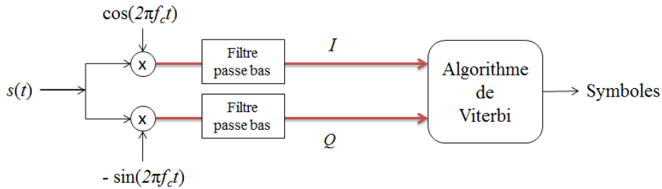
Figure 2.26 Chaîne de démodulation.
