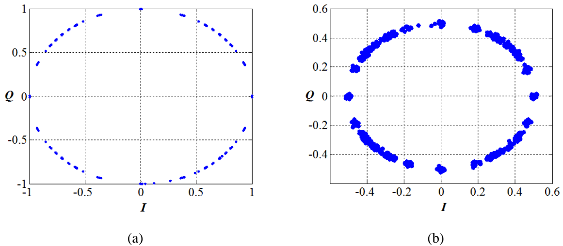
Figure 3.4. Constellations des signaux en quadrature I(nTe) et Q(nTe) , a : avant canal BBAG , b : après canal BBAG de SNR = 30 dB, avec un pas d'échantillonnage de 4 échantillons par symbole (en simulation).
