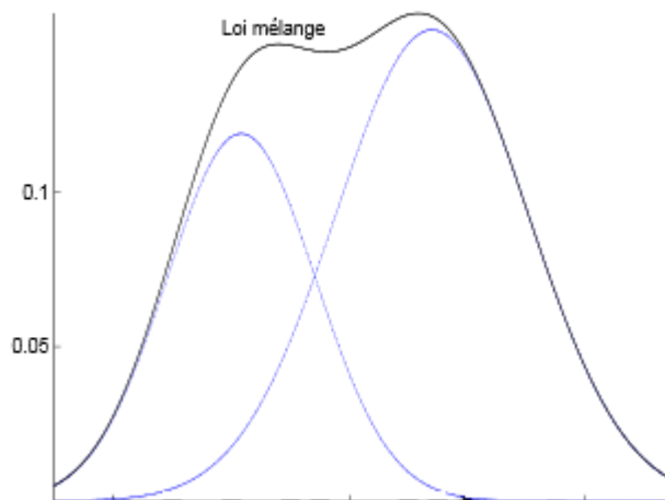
Figure 3.15. Mélangement multi gaussien (2 gaussiennes).
