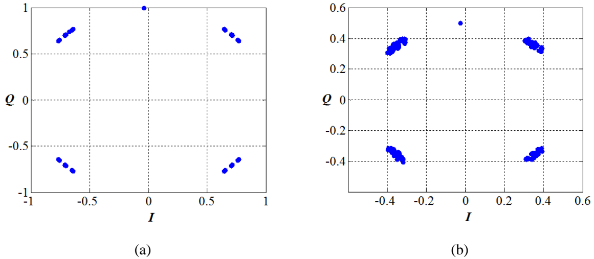
Figure 3.3. Constellations des signaux en quadrature I(nTe) et Q(nTe) , a : avant canal BBAG , b : après canal BBAG de SNR = 30 dB, avec un pas d'échantillonnage de 1 échantillon par symbole (en simulation).
