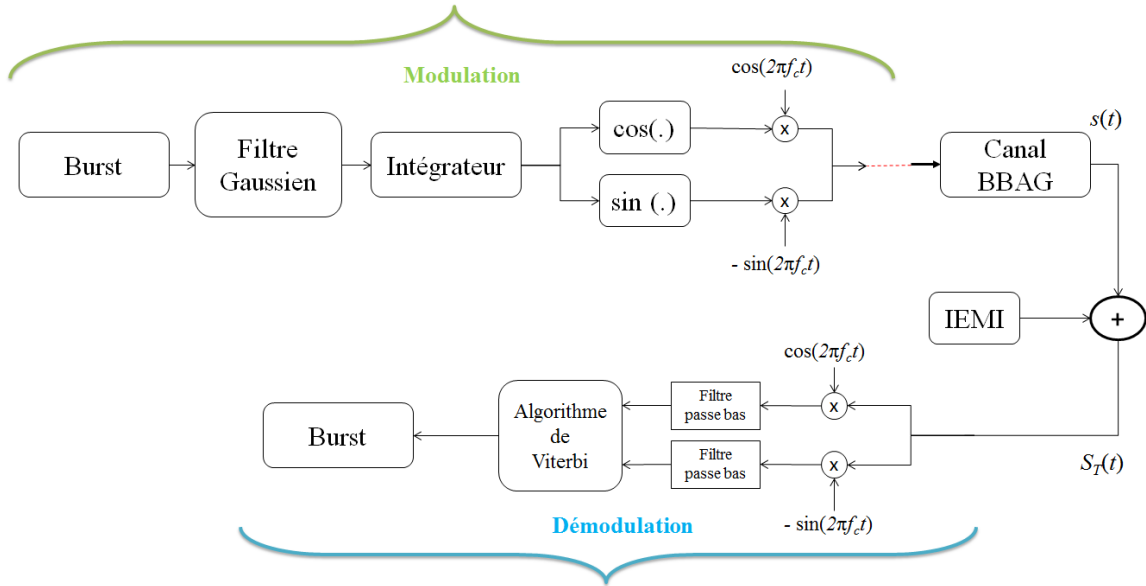
Figure 2.24 Chaîne de modulation / démodulation GSMK.
