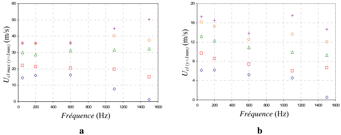
Figure 3.17 - Variation de la vitesse axiale avec la fréquence du JS pour y=1mm et pour plusieurs amplitudes de pression a) vitesse maximum, b) vitesse moyenne A = \diamond : 250 Pa, \square : 500 Pa, \triangle : 1000 Pa, \circ : 1500 Pa, + : 2000 Pa
