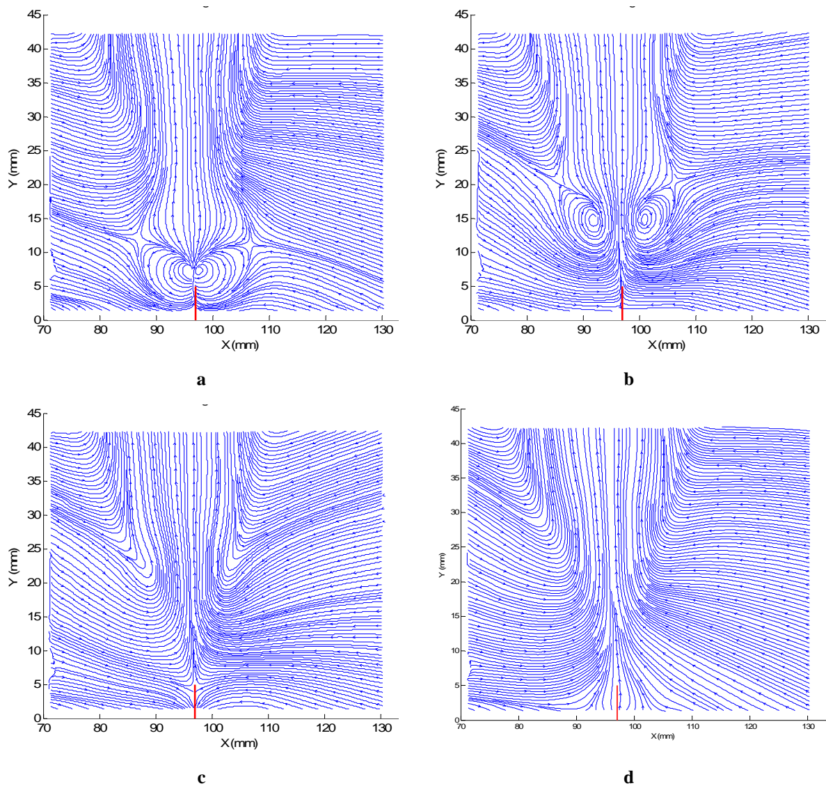
Figure 3.23 – Lignes de courant pour le JS à 4 instants correspondant à : a. t/T = 0.25 , b. t/T = 0.5 , c. t/T = 0.75 , d. t/T = 1 - f = 200 \text{ Hz} , A = 2000 \text{ Pa}
