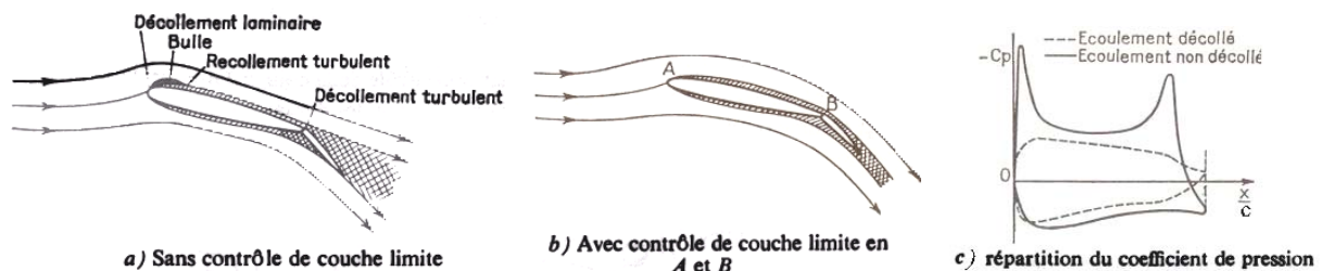
Figure 1.42 – Écoulement autour d'une aile aux grands angles d'incidence [1]
