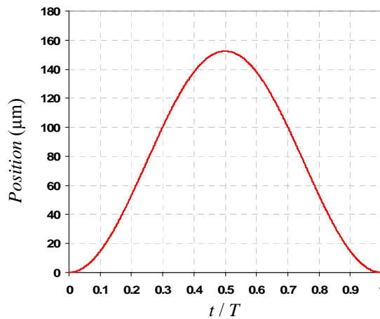
Figure 3.3 –Variation de la position de la membrane du JS avec le temps
