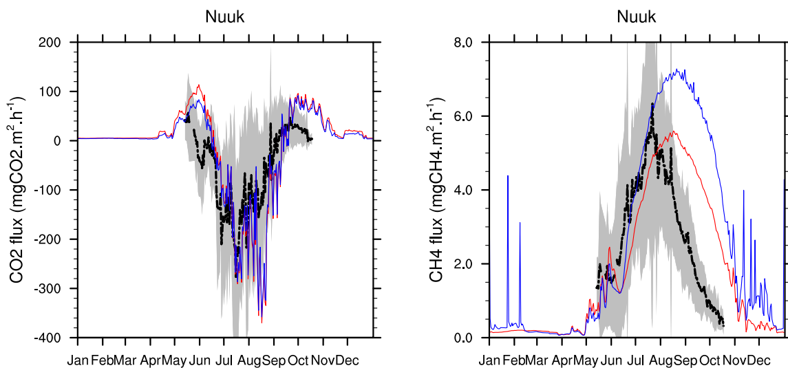
FIGURE 4.23 – Profils de carbone du sol (haut) et flux de gaz à effets de serre observés et simulés après 8000 ans de spin-up, une advection de 1 \text{ mm.an}^{-1} stoppée en dessous de 1m et des taux de décomposition multipliés par 5.
