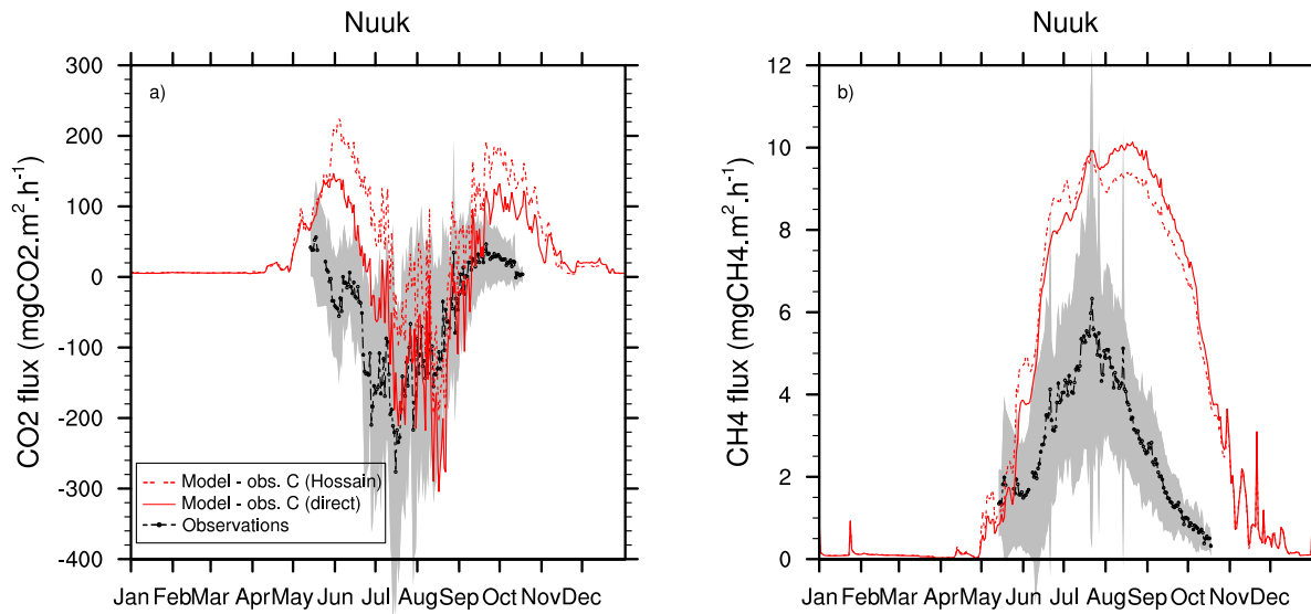
FIGURE 4.18 – Moyenne annuelle des flux journaliers de CO_2 (droit) et de CH_4 (gauche) observés, et simulés par le modèle forcé avec les profils de carbone observés (direct et indirects)
