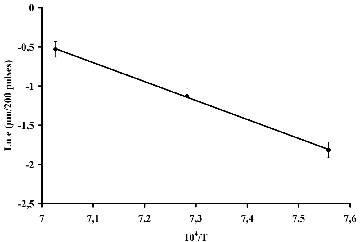
Figure VI.16 : Diagramme d'Arrhénius correspondant à n_p^{\text{TiC}}=200 .
