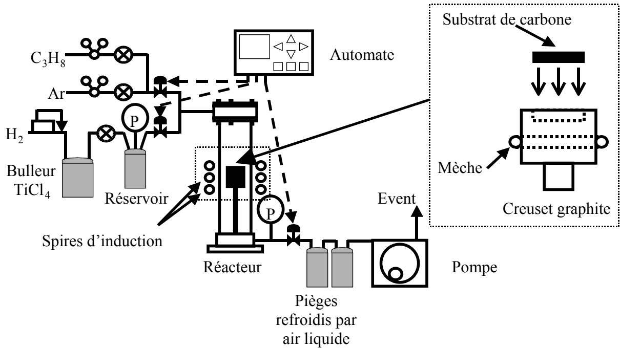
Figure IV.3 : Dispositif expérimental utilisé pour la P-CVD de PyC et la P-RCVD de TiC_x sur substrats de carbone.
