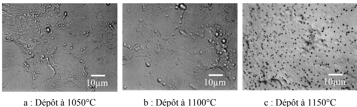
Figure IV.7 : Observation, par microscopie optique, de surfaces de dépôts PyC à différentes températures. Mise en évidence d'un phénomène de nucléation pour T = 1150^\circ\text{C} .
