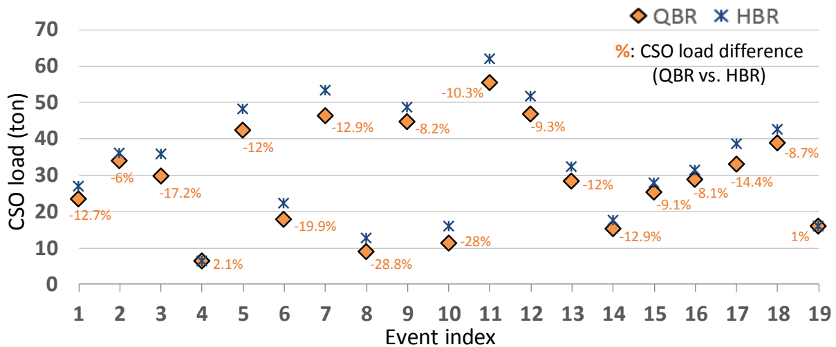
Figure 5. Charges totales des CSO obtenues par les deux stratégies pour les 19 événements sélectionnés, ainsi que la différence de charge des CSO entre le QBR et le HBR, en pourcentage.
