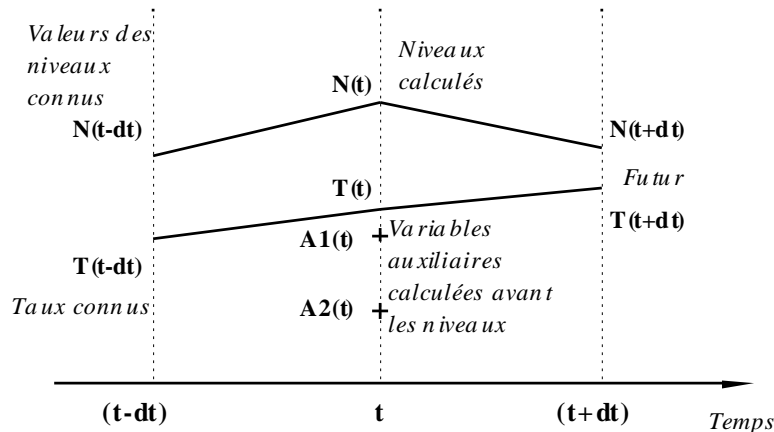
FIG 3 Principe de calcul DYNAMO
