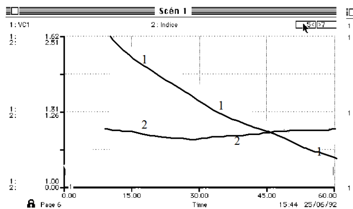
FIG 6 Scénario 1: Indice et service(t)
