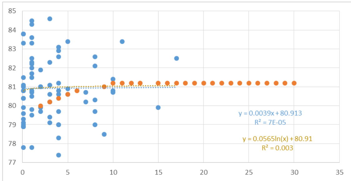
Figure 60 Mesures en bleu de LAmx sur revêtements R3 de la base de données de l'ex-LRPC de Strasbourg, tests de corrélations à l'âge du revêtement en bleu clair et jaune, et modèle NMPB en orange (formes de régression sur mesures (points bleus) en pointillés, et leur extrapolation jusqu'à t=30 ans sous forme de points). En ordonnée : niveau sonore (dB(A)) ; en abscisse : âge du revêtement (ans).
