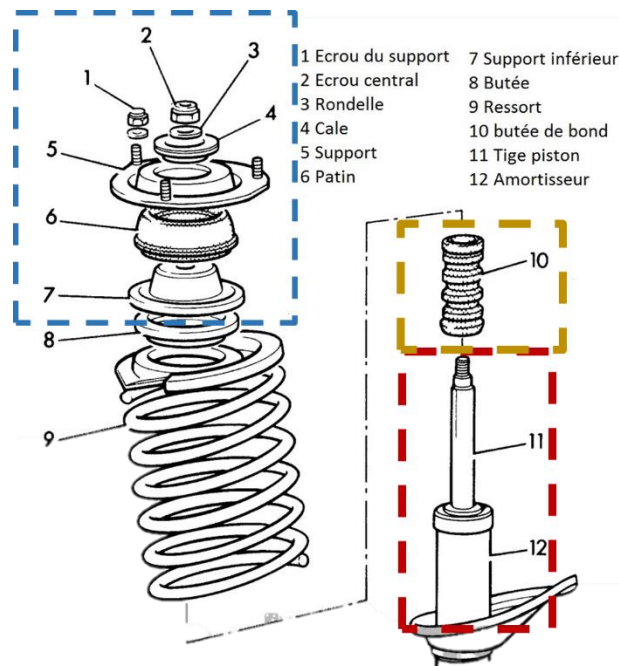
Figure 76 Schéma d'un kit complet d'amortisseur hydraulique et identification des pièces d'usure (bleu : tête d'amortisseur ; jaune : butée ; rouge : vérin)
