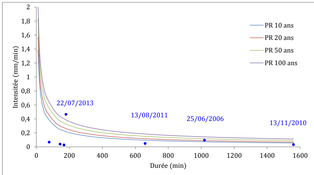
Figure 2.53 - Représentation des évènements retenus sur le diagramme intensité-durée-fréquence (IDF) local (Courbe IDF tracé à partir des coefficients de MONTANA de la station Météo France de Caen-Carpiquet).
