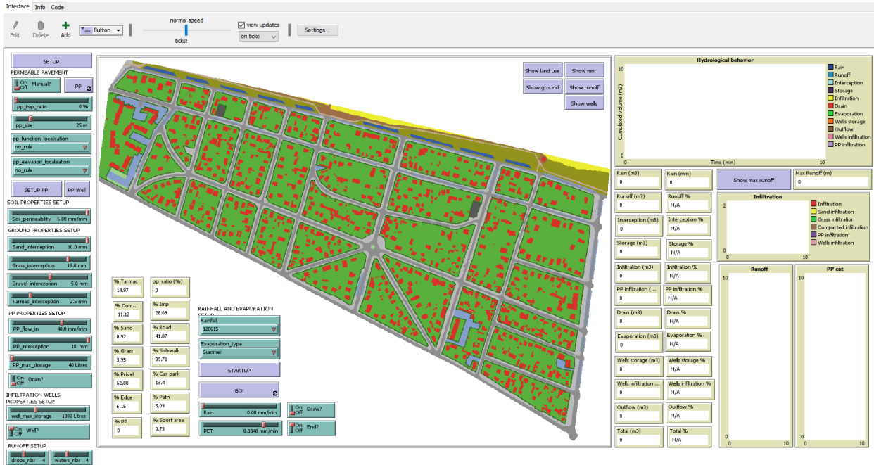
Figure 4.2 - Visualisation de l'interface graphique du modèle PorousCity . En gris, les boutons, en vert les objets qui permettent de définir des données d'entrée, en jaune les sorties du modèle sous forme numérique ou graphique, enfin la zone au centre est l'espace de visualisation du domaine de modélisation.
