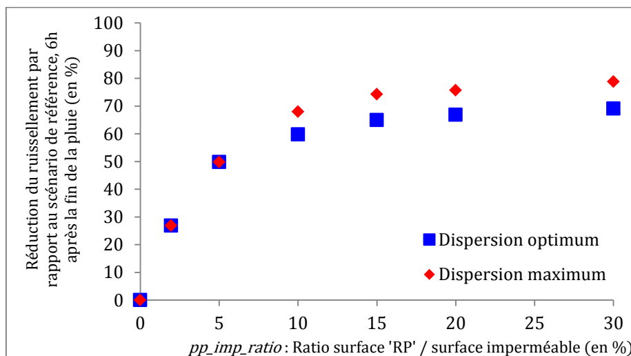
Figure 4.57 – Réduction du ruissellement exprimé en pourcentage du volume de ruissellement du scénario de référence, tracé en fonction du ratio de surface de RP sur la surface imperméable.
