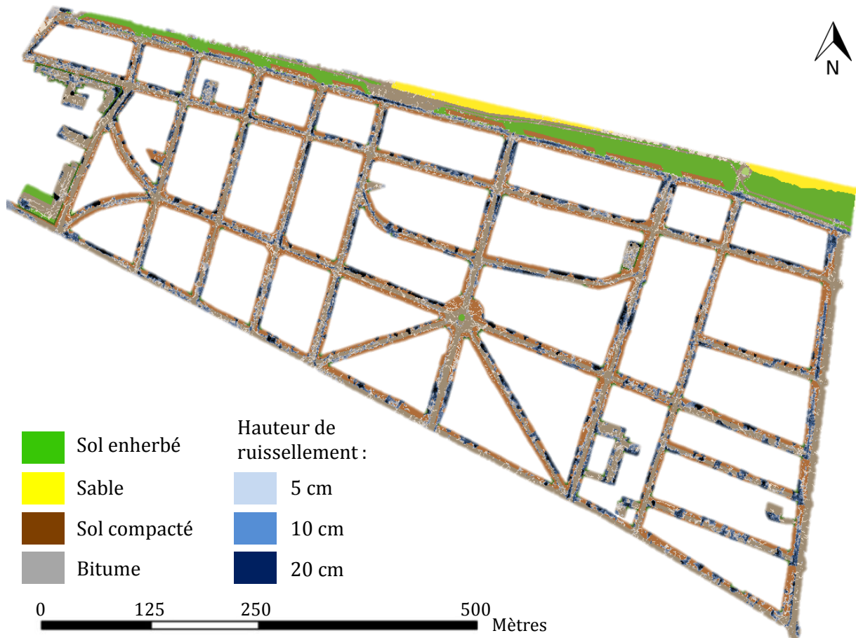
Figure 4.36 – Sortie du modèle PorousCity . Visualisation de la hauteur d'eau sur les cellules actives au moment de la fin de la pluie (volume de ruissellement maximum). Simulation de la pluie du 11/06/2015 avec K_s = 1 \cdot 10^{-5} m/s
