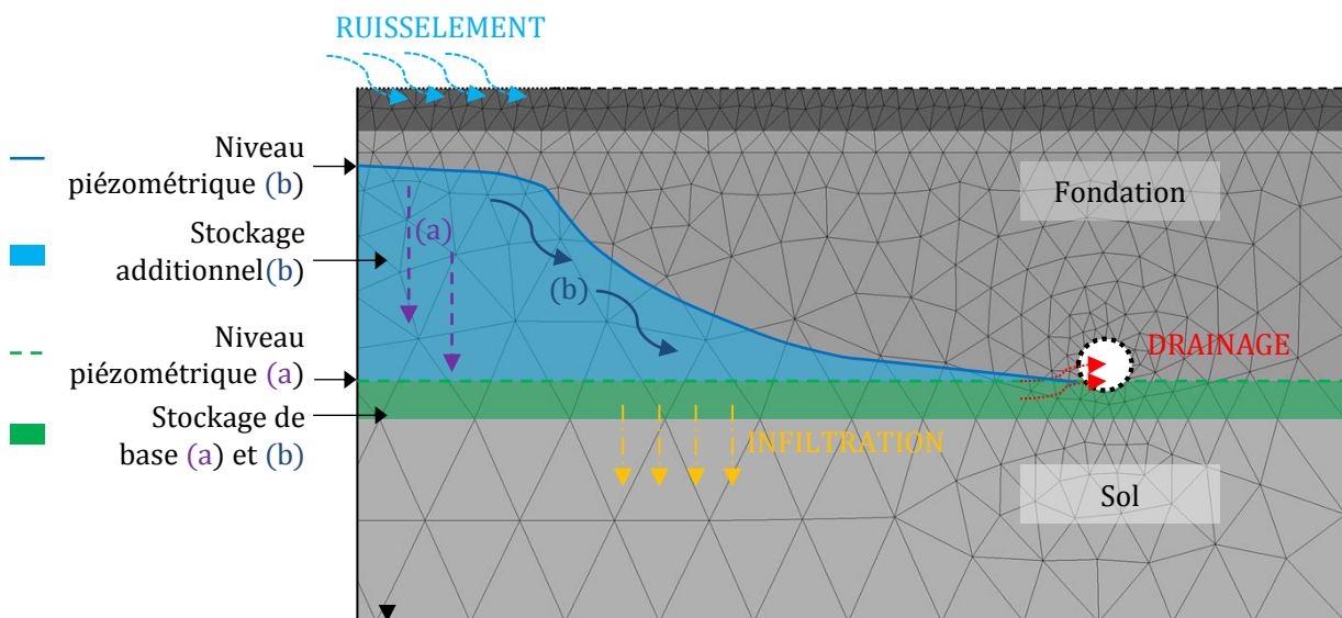
Figure 3.37 – Schéma d’illustration de l’influence de K_s (fondation) sur le stockage dans la structure au moment du pic de stockage. (a) K_s (fondation) = 0,1 m/s et (b) K_s (fondation) = 0,001 m/s
