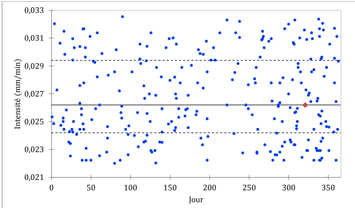
Figure C.12 - Nuage de points de la typologie "évènements faibles". Représentation des 1 er et 3 ème quartiles, de la médiane et de l'évènement retenu
