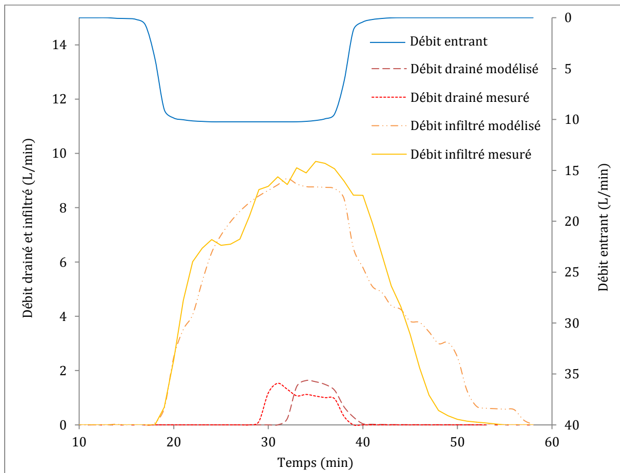
Figure 3.26 – Comparaison des hydrographes modélisés et mesurés (échelle de gauche) et visualisation du débit en entrée (échelle de droite). Essai de vérification b2.
