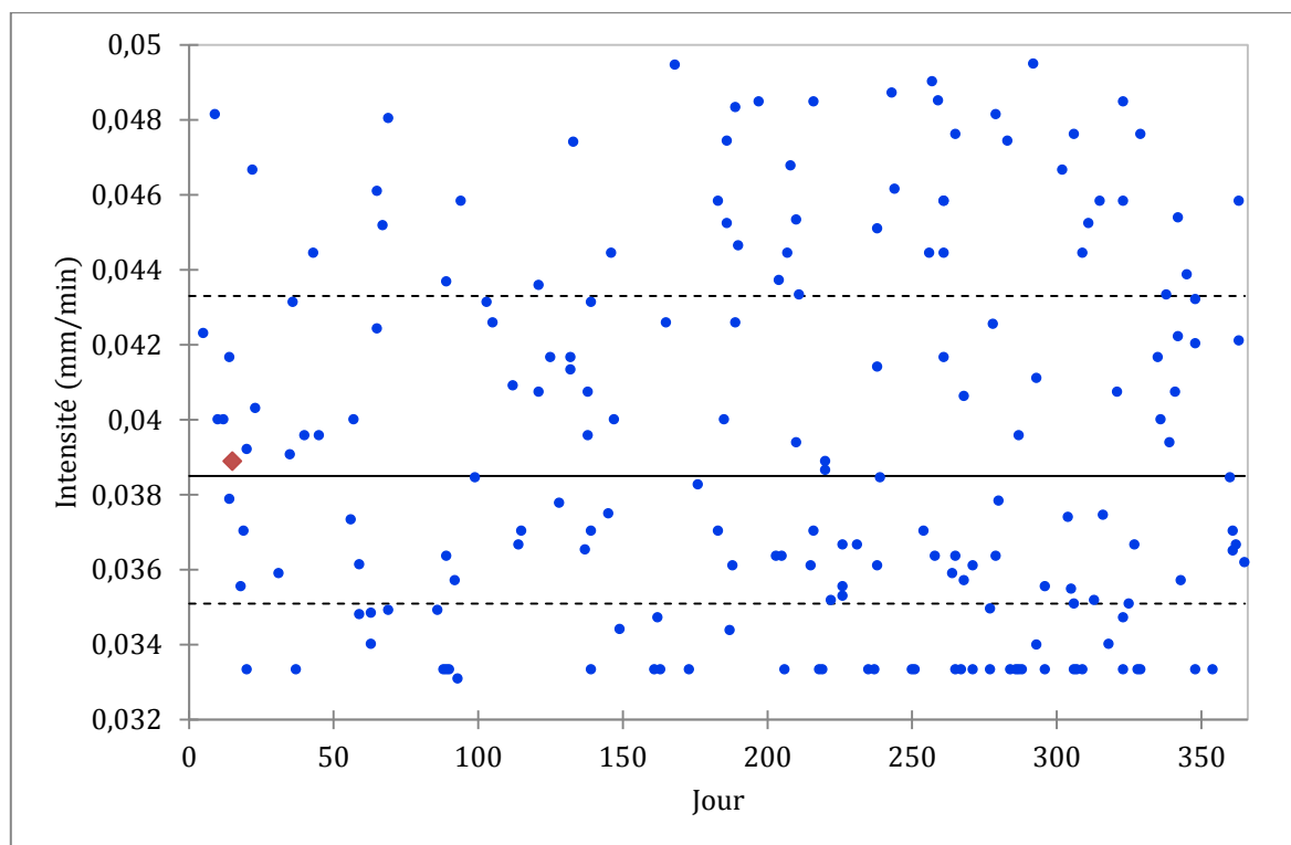
Figure C.10 - Nuage de points de la typologie "évènements courants". Représentation des 1 er et 3 ème quartiles, de la médiane et de l'évènement retenu
