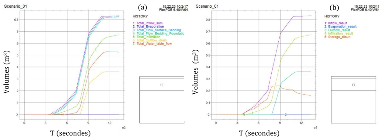
Figure 3.16 – Sorties du modèle PermetAble . Évolution des volumes en entrée et sortie de chaque couche (a), et des indicateurs hydrologiques (b) (Scénario de référence).
