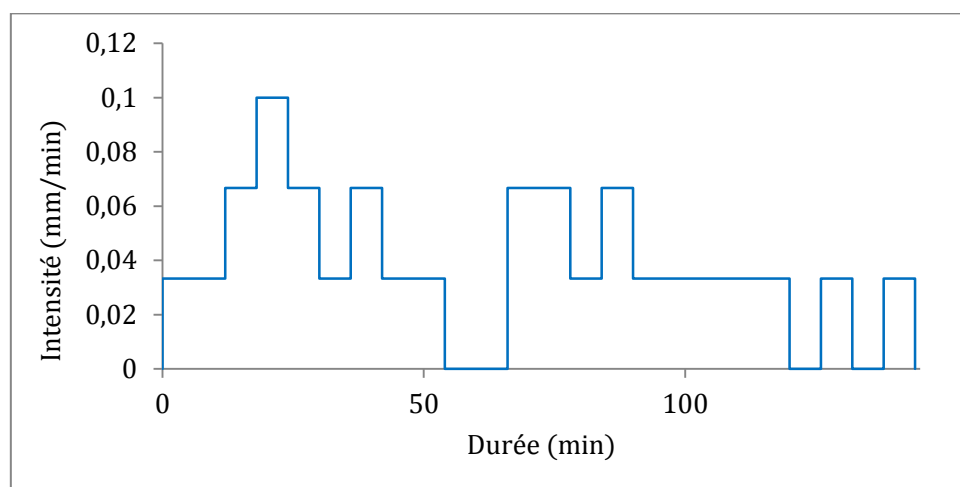
Figure C.11 - Évènement pluviométrique du 15/01/2008
