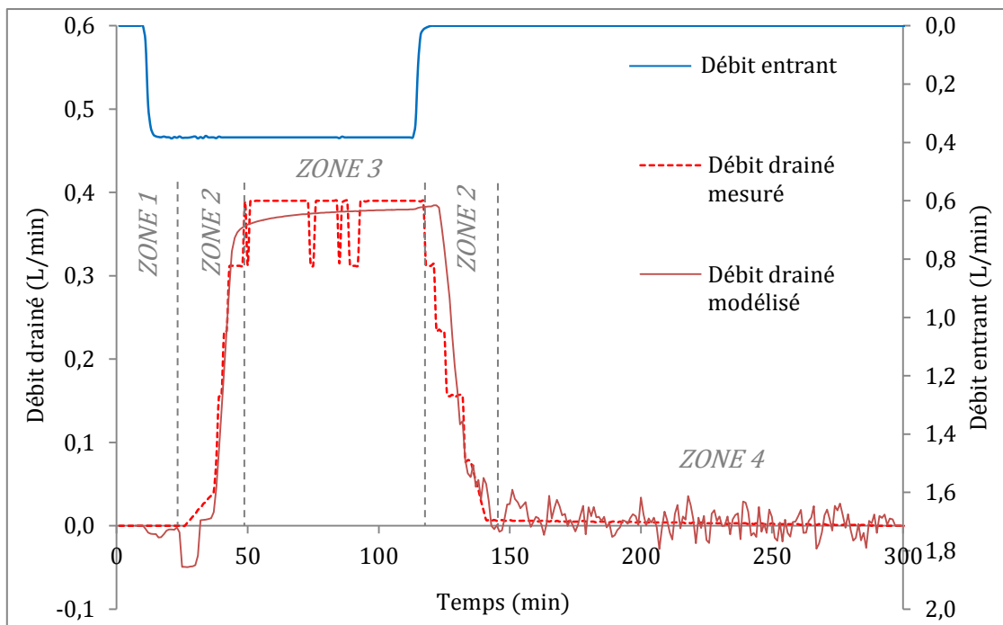
Figure 3.22 – Comparaison entre les hydrographes des débits drainés mesurés et simulés (échelle de gauche) et représentation de l'hydrographe du débit en entrée (échelle de droite) (essai de calage du modèle PermetAble )
