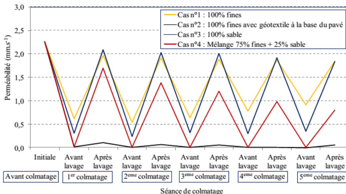
Figure B.2 - Variation de la perméabilité des bétons drainants classiques en fonction du type de matériaux de colmatage (Nguyen, 2014)
