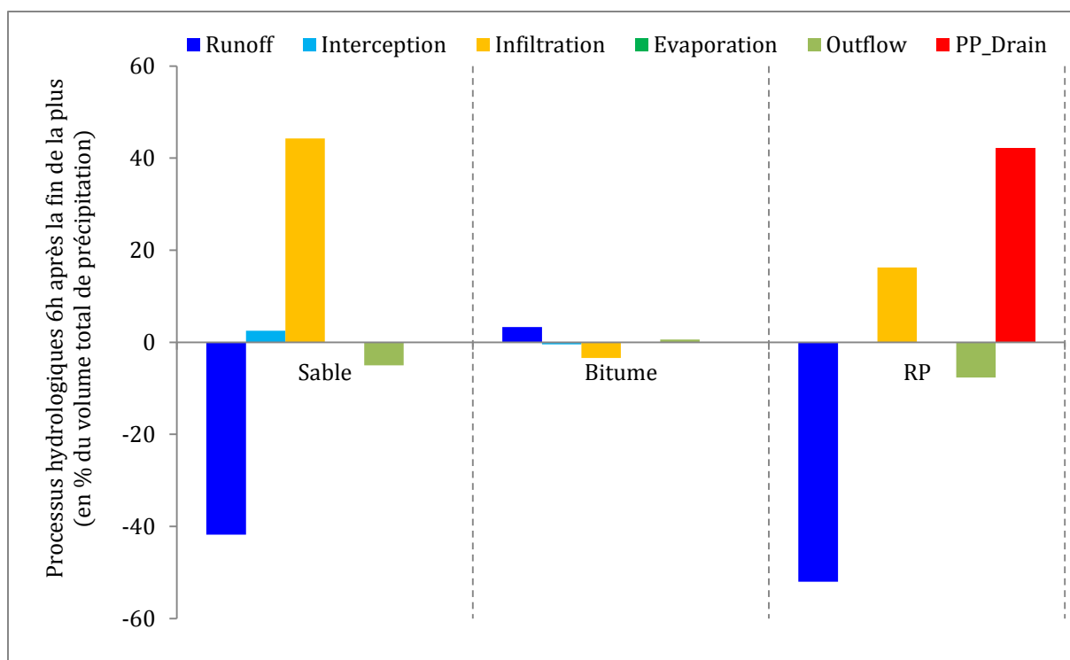
Figure 4.44 – Écarts de volume des processus hydrologiques des trois scénarios 'trottoirs' avec le scénario 'référence' (résultats exprimés en % du volume total de précipitation).
