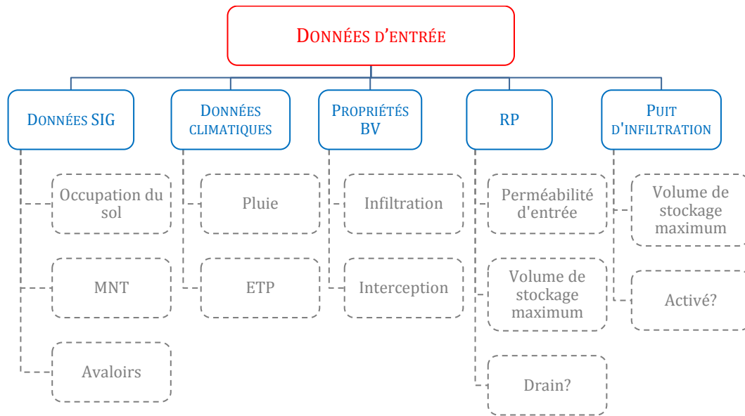
Figure 4.13 - Schématisation des données d'entrée du modèle PorousCity
