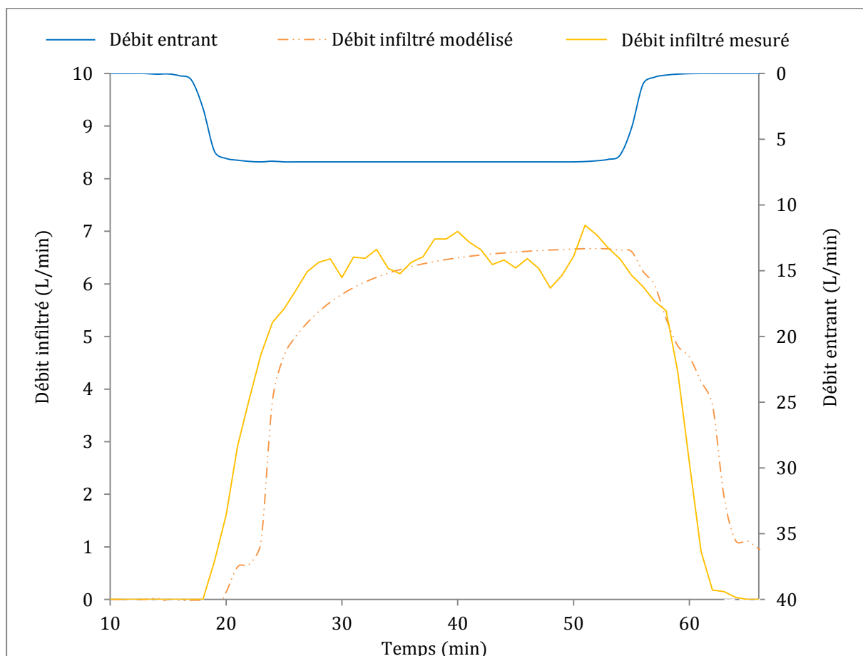
Figure 3.24 - Comparaison des hydrographes d'infiltration modélisés et mesurés (échelle de gauche) et visualisation du débit en entrée modélisé (échelle de droite). Essai de vérification b1.
