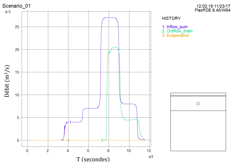
Figure 3.39 – Sortie du modèle PermetAble . Visualisation des débits entrants et évacués par le drain au cours du temps. Graphique exporté à la fin de la pluie (Scénario de référence).
