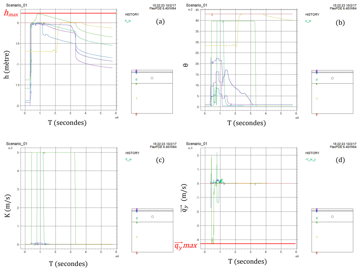
Figure 3.15 - Sorties du modèle PermetAble . Visualisation des variations de h (a), θ (b), K (c) et \vec{q}_y (d) en fonction du temps le long de la coupe 1 (Scénario de référence). Représentation de h max et de \vec{q}_y maximum.
