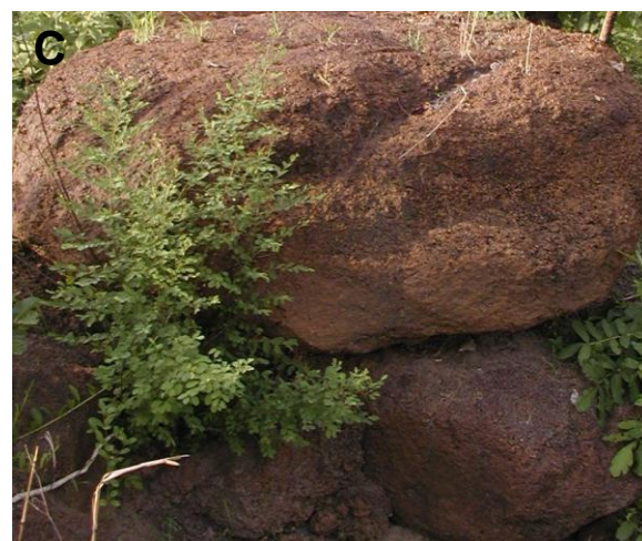
Gros blocs de cuirasses latéritiques. Souvent sous forme de graviers épars, de dalles ou de gros blocs (comme sur cette image), les cuirasses constituent une formation superficielle prépondérante sur le bassin d'Ara.
