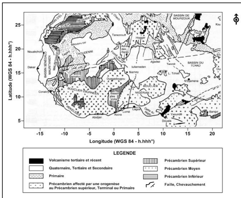
Figure 3: Esquisse géologique de l'Afrique de l'ouest (Fabre, 1971).
